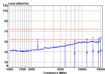
BT_DH5_TX_CH_39_Horizontal
