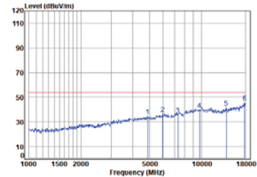
Right BLE_2M_TX_CH_19_Horizontal-Avg
