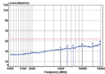
Left BLE_2M_TX_CH_38_Horizontal-Avg
