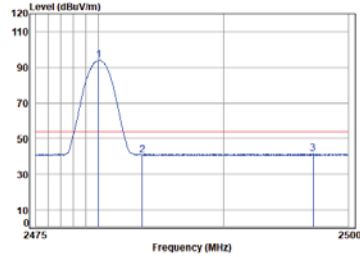
Left BLE_1M_TX_CH_39_Horizontal-Avg
