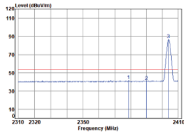
Left BLE_2M_TX_CH_01_Vertical-Avg
