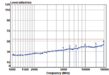
Right BLE_2M_TX_CH_38_Horizontal-Avg
