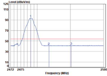
Left BLE_2M_TX_CH_38_Horizontal-Avg
