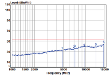
Right BLE_2M_TX_CH_01_Horizontal-Avg
