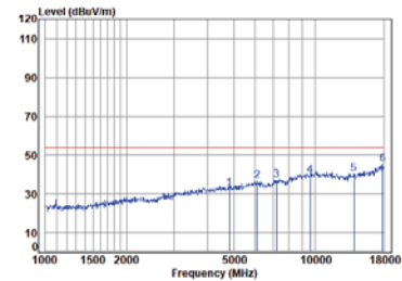
Right BLE_2M_TX_CH_01_Vertical-Avg
