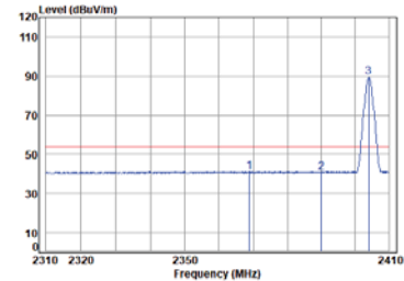
Right BLE_2M_TX_CH_01_Horizontal-Avg
