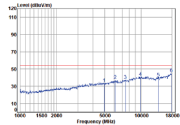
Right BLE_2M_TX_CH_38_Vertical-Avg
