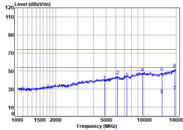
Right BT_DH5_TX_CH_39_Horizontal
