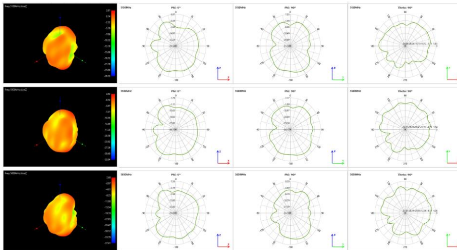
ANT4 WIFI5.8G L=105MM红 方向图
