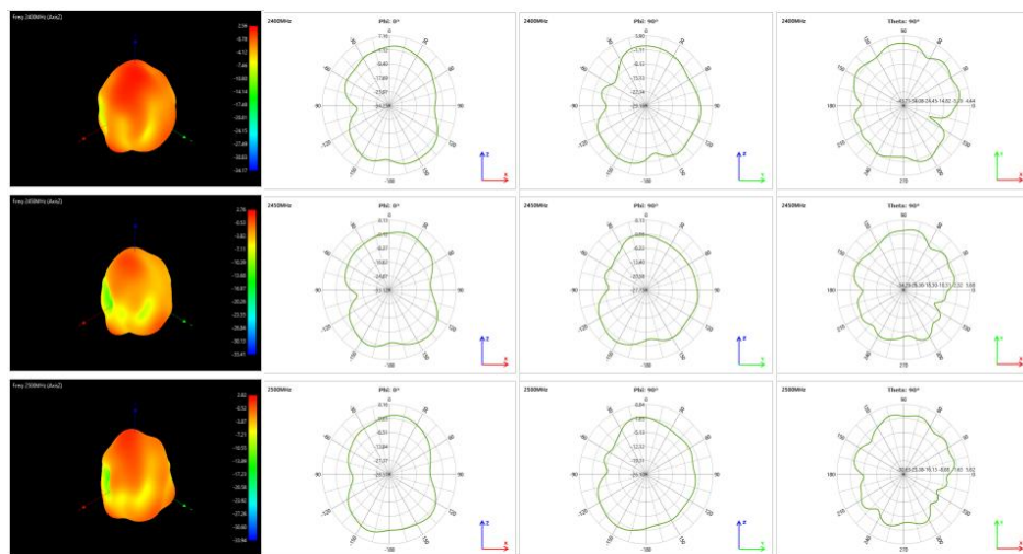
ANT2 WIFI 2.4G L=305MM黑 方向图
