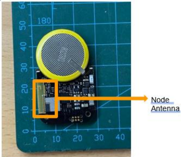
Fig A3: Node Antenna highlighted
