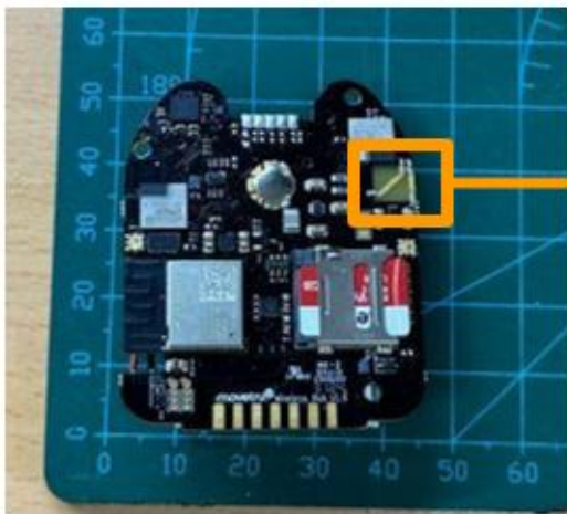
Fig A6: Hub Antenna highlighted
