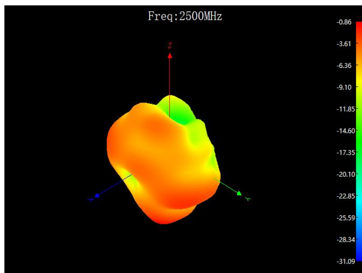
2500MHz 3D
