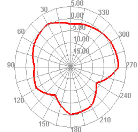
2450.000MHz E2
