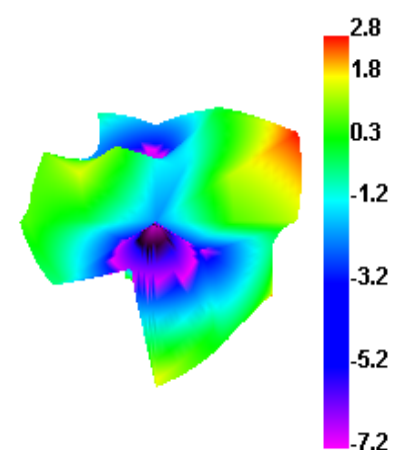
2430.000MHz E1
