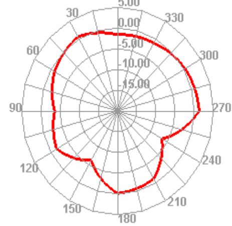
2440.000MHz H
