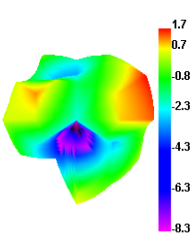
2400.000MHz E1
