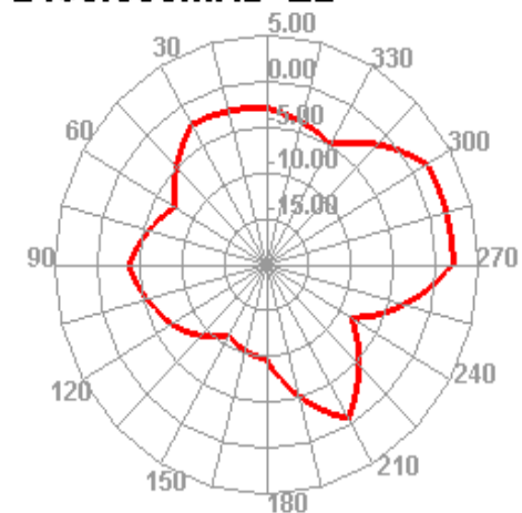
2470.000MHz H
