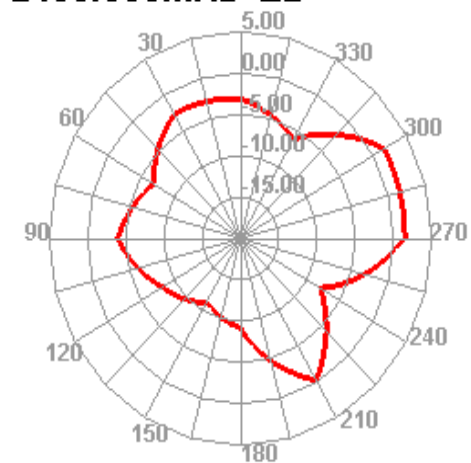
2450.000MHz E2
