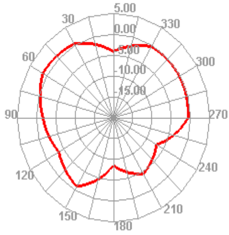
2410.000MHz
