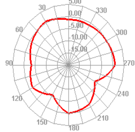
2430.000MHz E2
