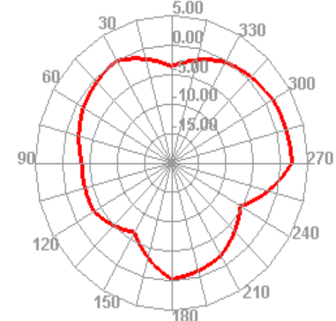
2470.000MHz H
