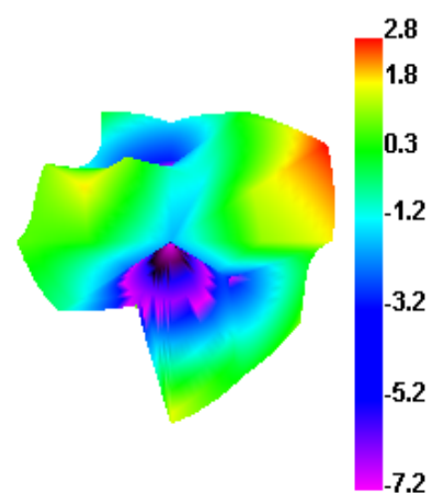
2420.000MHz E1
