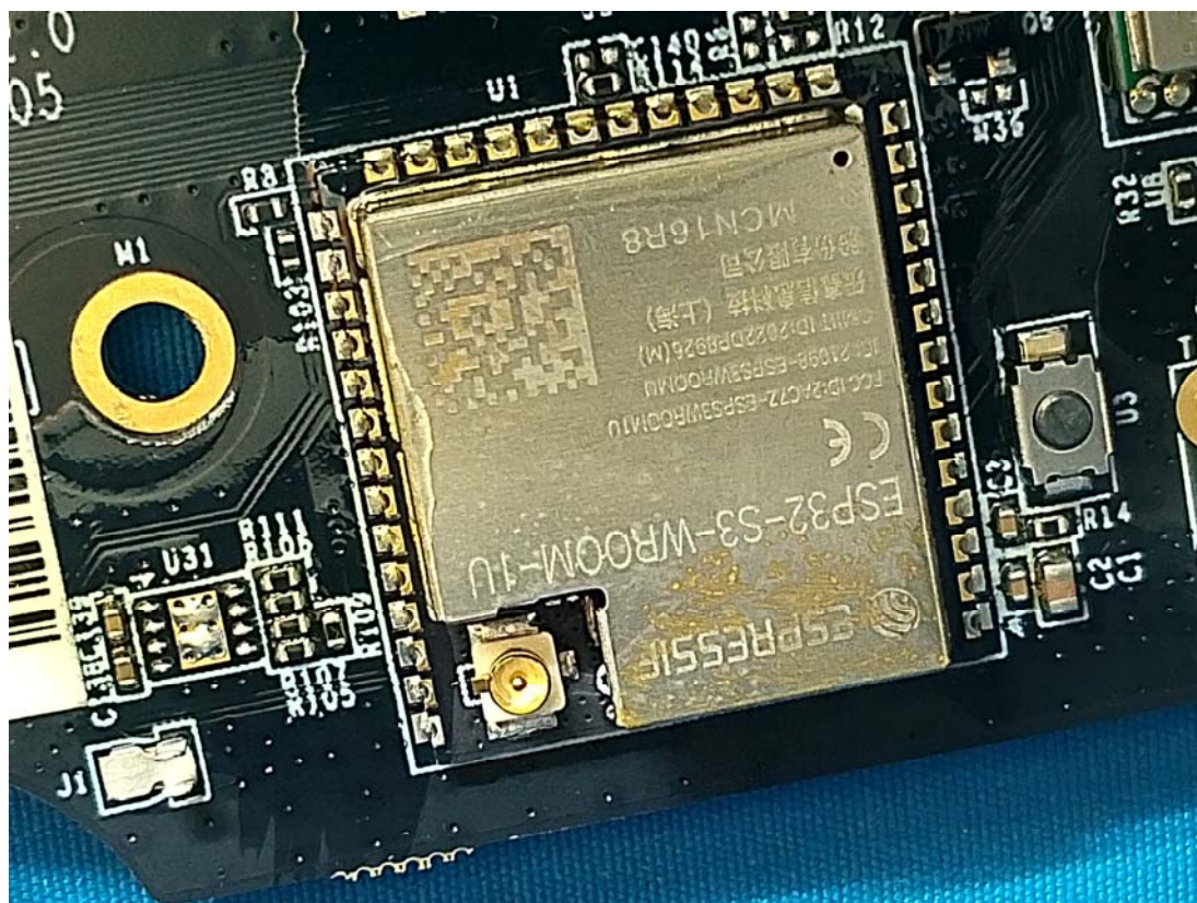
2.4G Wifi Module
