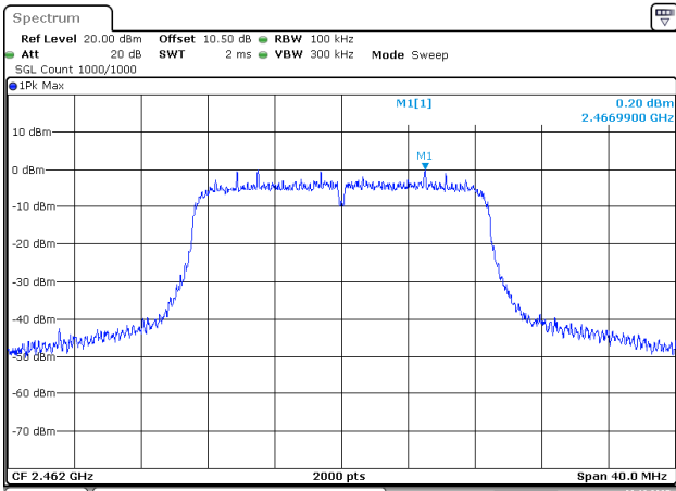
802.11n20_2462MHz
