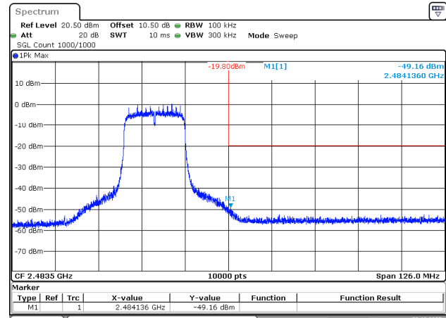
802.11n20_2462MHz
