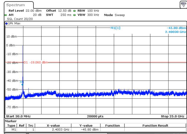
802.11n20_2437MHz
