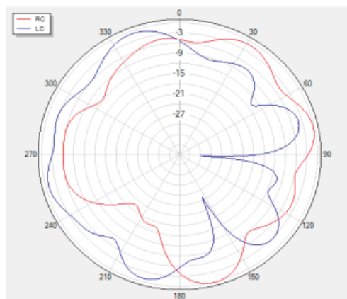
Theta=90 freq=2400MHz
