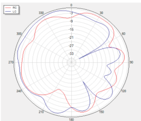
Theta=90 freq=2500MHz
