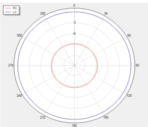
Theta=0 freq=2500MHz
