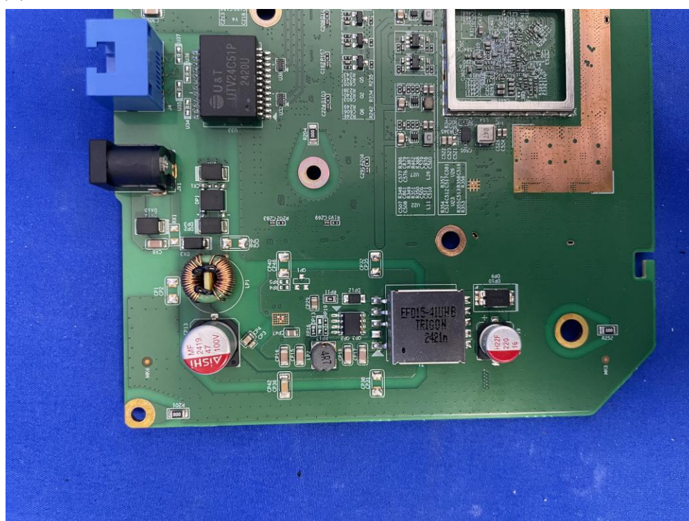
(8) EUT Photo
