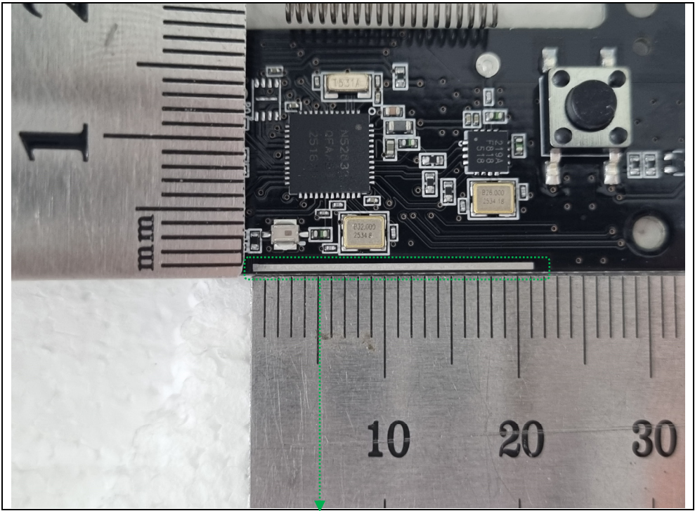
<BLE antenna>
