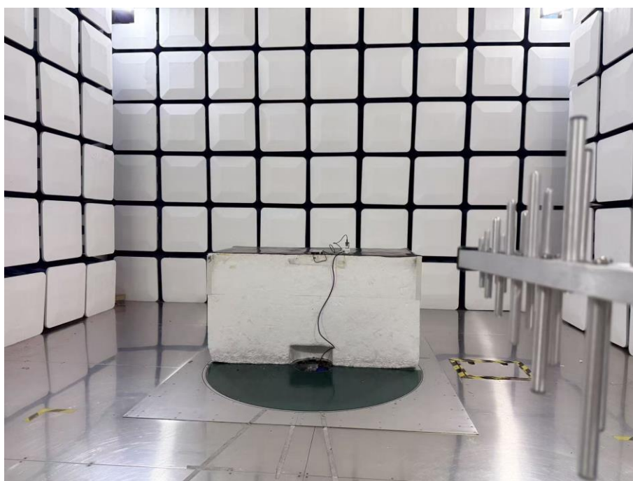
30MHz-1GHz-RFID
