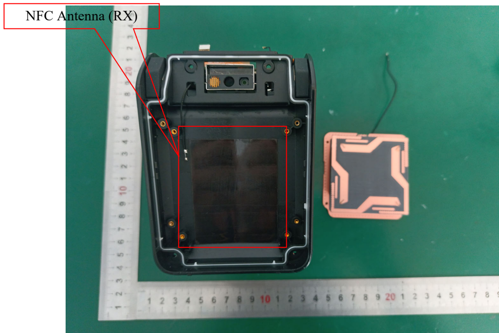
RFID Antenna
