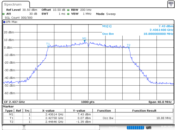
802.11ax20_2437MHz_Chain 0
