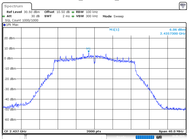
802.11n20_2437MHz_Chain 1
