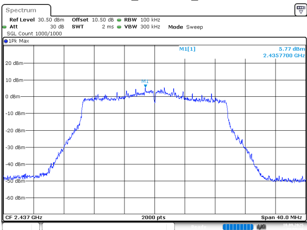
802.11ax20_2437MHz_Chain 0
