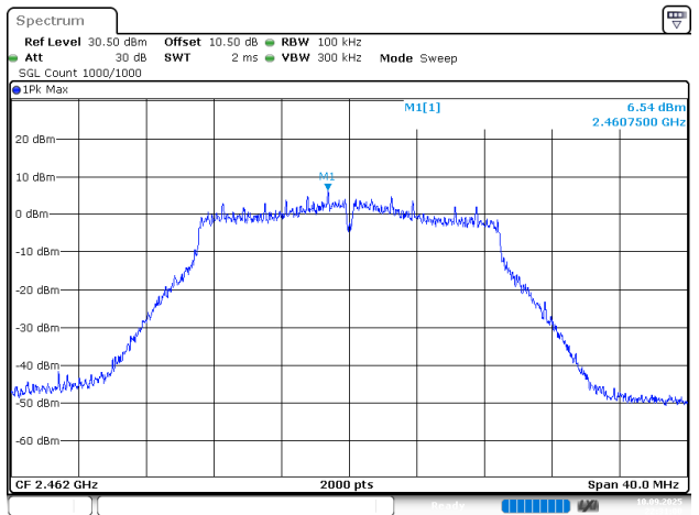
802.11n20_2462MHz_Chain 1
