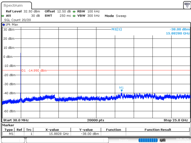
802.11ax20_2462MHz_Chain 0
