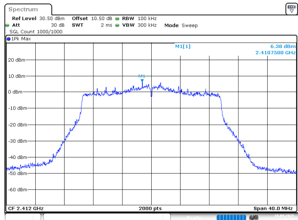
802.11ax20_2412MHz_Chain 1
