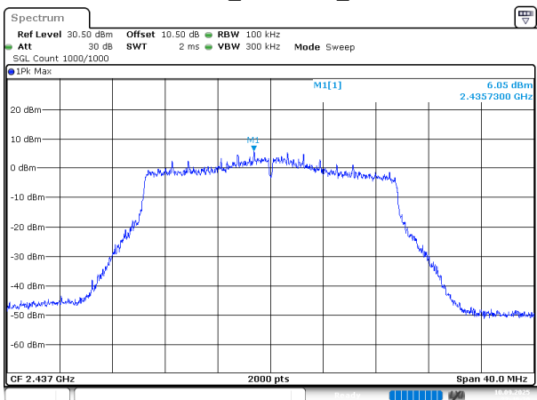
802.11ax20_2437MHz_Chain 1
