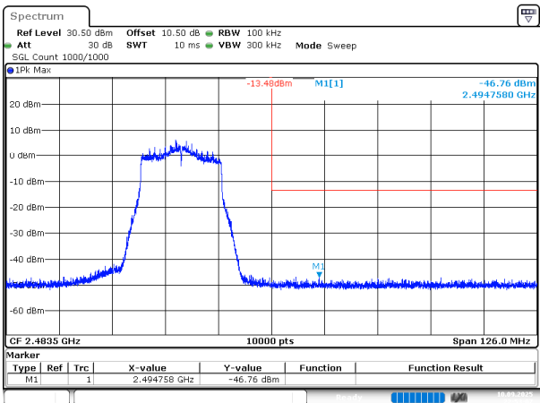
802.11ax20_2462MHz_Chain 1
