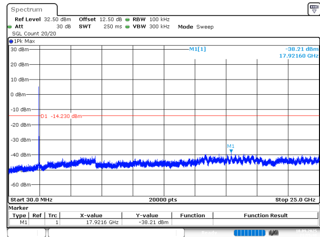
802.11ax20_2437MHz_Chain 0
