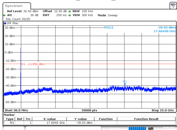
802.11ax20_2437MHz_Chain 1
