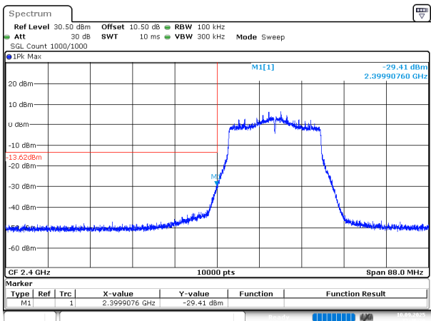
802.11ax20_2412MHz_Chain 1
