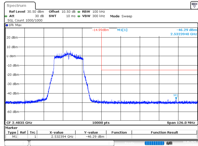
802.11ax20_2462MHz_Chain 0
