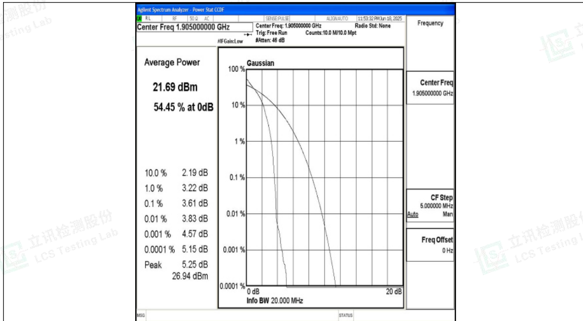
Band25-20MHz-QPSK-26590-1RB#0-PASS
