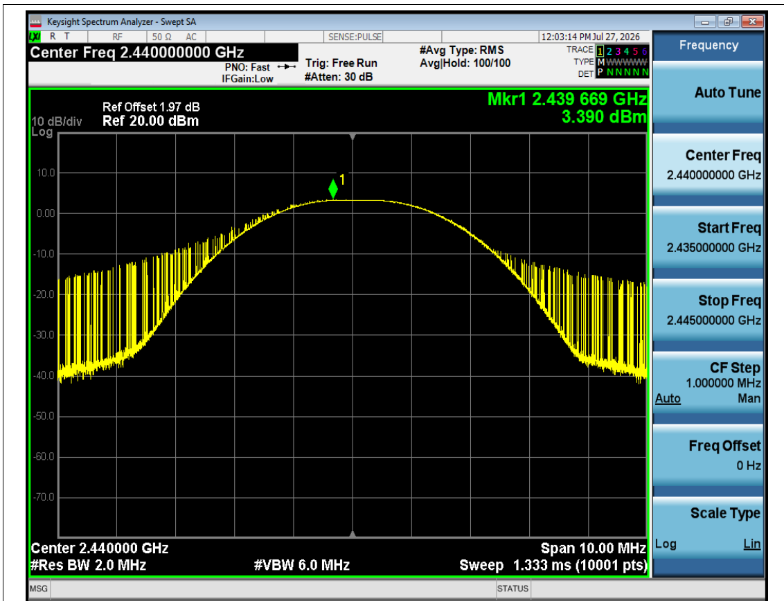
Peak Power NVNT BLE 2M 2440MHz Ant1
