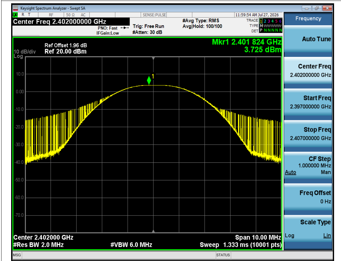
Peak Power NVNT BLE 2M 2402MHz Ant1
