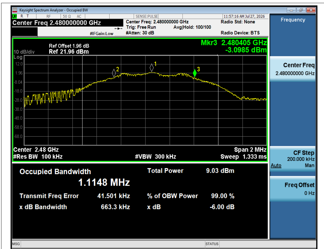
-6dB Bandwidth NVNT BLE 1M 2480MHz Ant1
