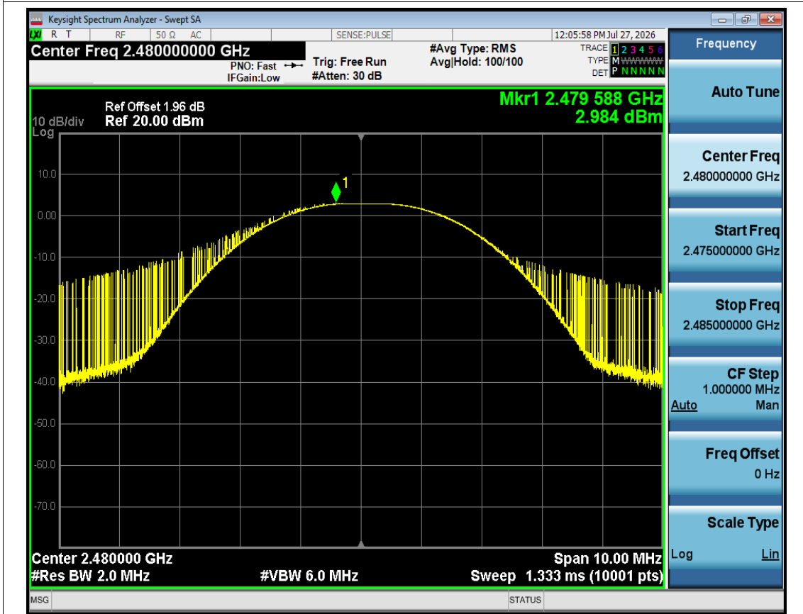
Peak Power NVNT BLE 2M 2480MHz Ant1
