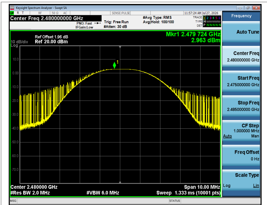
Peak Power NVNT BLE 1M 2480MHz Ant1
