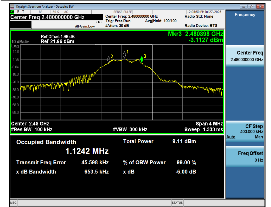
-6dB Bandwidth NVNT BLE 2M 2480MHz Ant1
