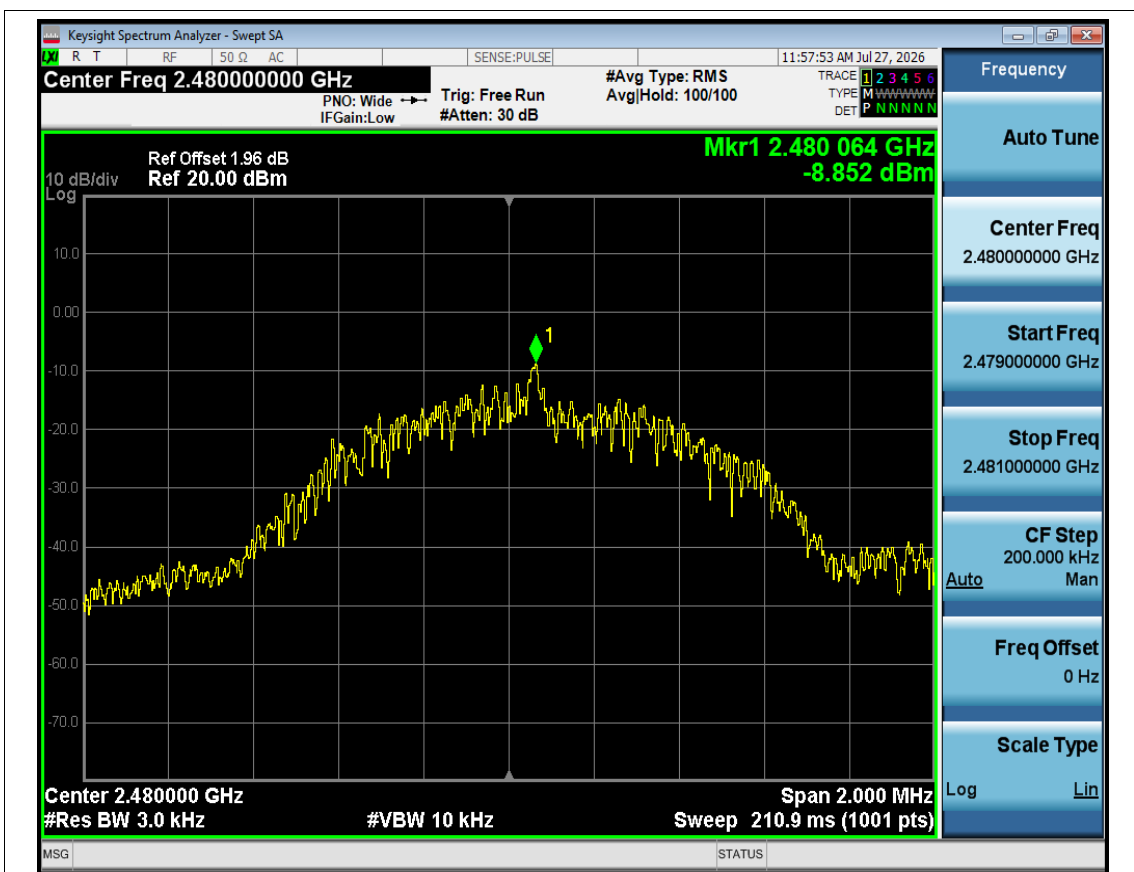
PSD NVNT BLE 1M 2480MHz Ant1
