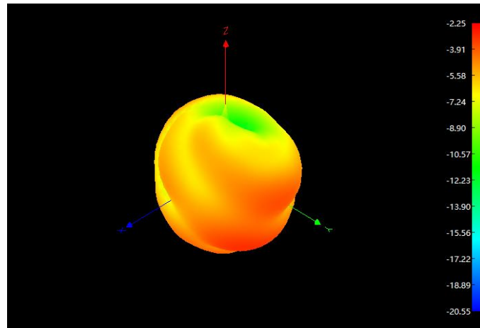
2500MHz 3D
