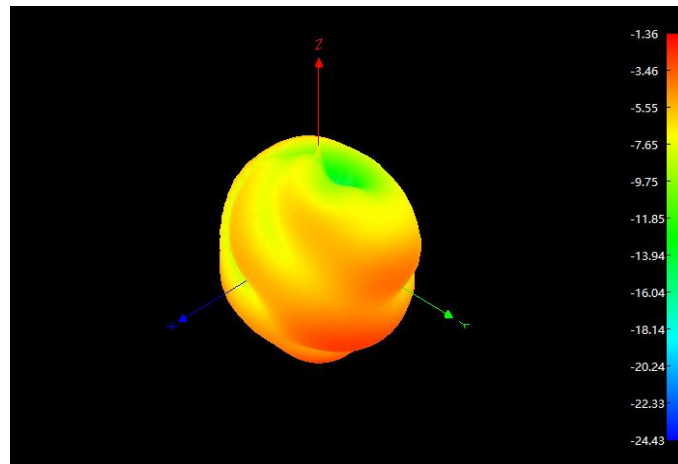
2450MHz 3D
