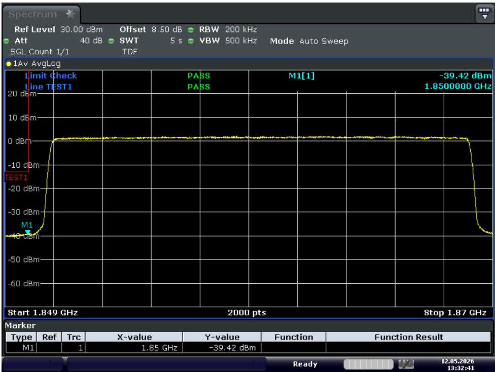
Test_Graph_band2_1860MHz_20M_16QAM_1RB#LOW_Band edge
