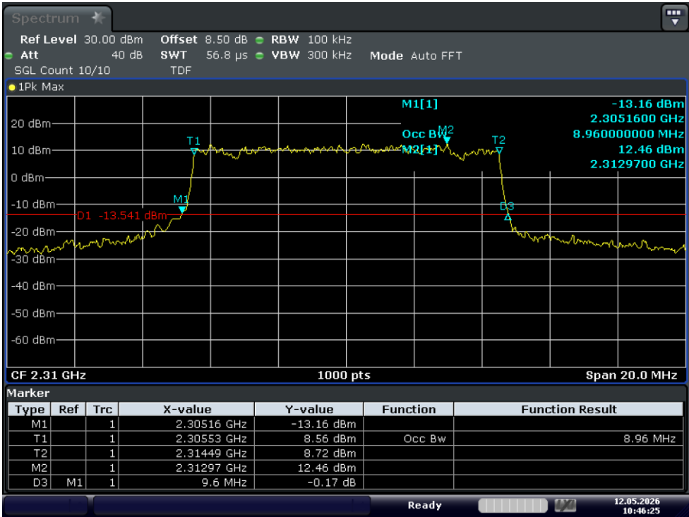
Test_Graph_band40(2305-2315)_2310MHz_10M_QPSK_50RB#LOW_OBW&EBW
