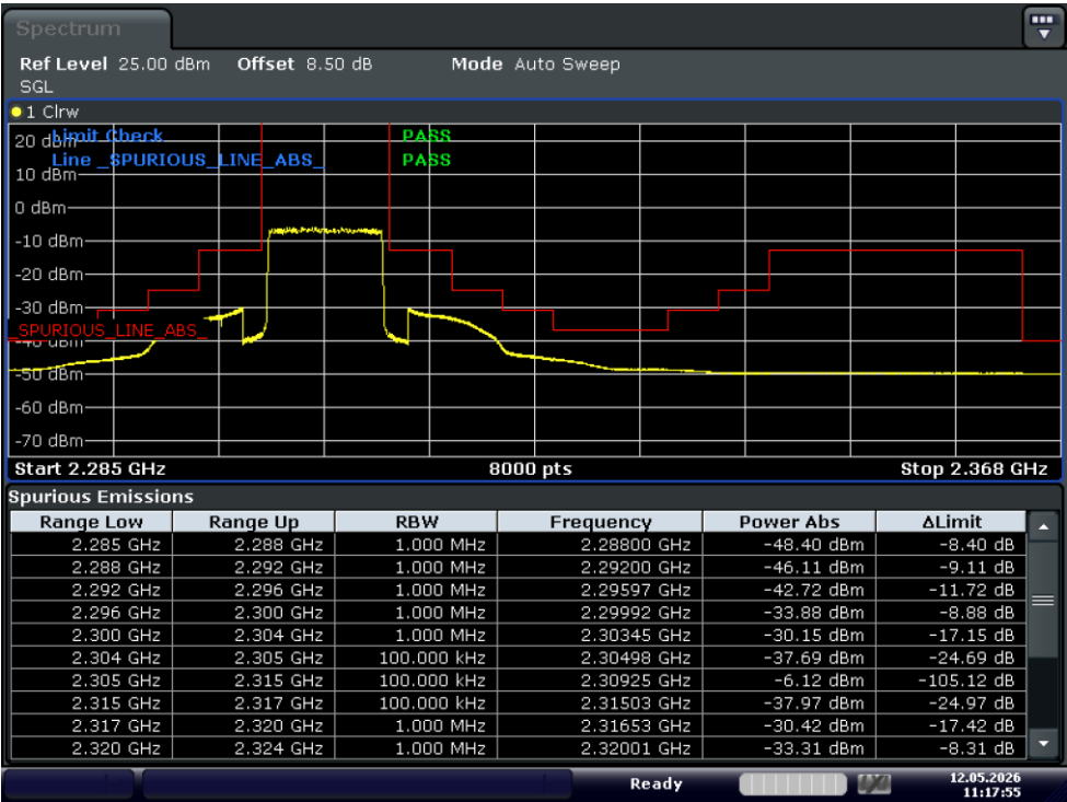
Test_Graph_band40(2305-2315)_2310MHz_10M_QPSK_50RB#LOW_Band edge
