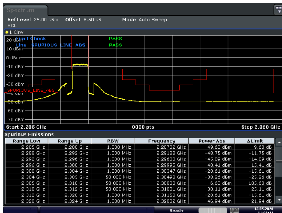
Test_Graph_band40(2305-2315)_2307.5MHz_5M_16QAM_1RB#LOW_Band edge
