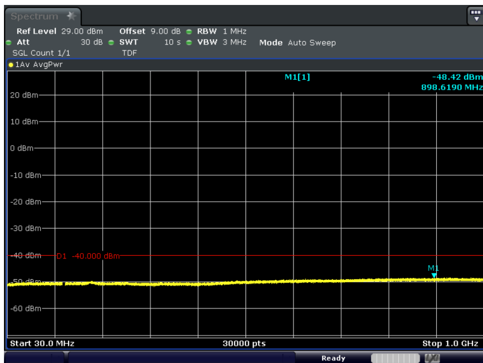
Test_Graph_band40(2305- 2315)_2307.5MHz_5M_QPSK_25RB#LOW_30M_1G_TX
