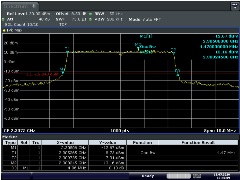
Test_Graph_band40(2305-2315)_2307.5MHz_5M_16QAM_25RB#LOW_OBW&EBW
