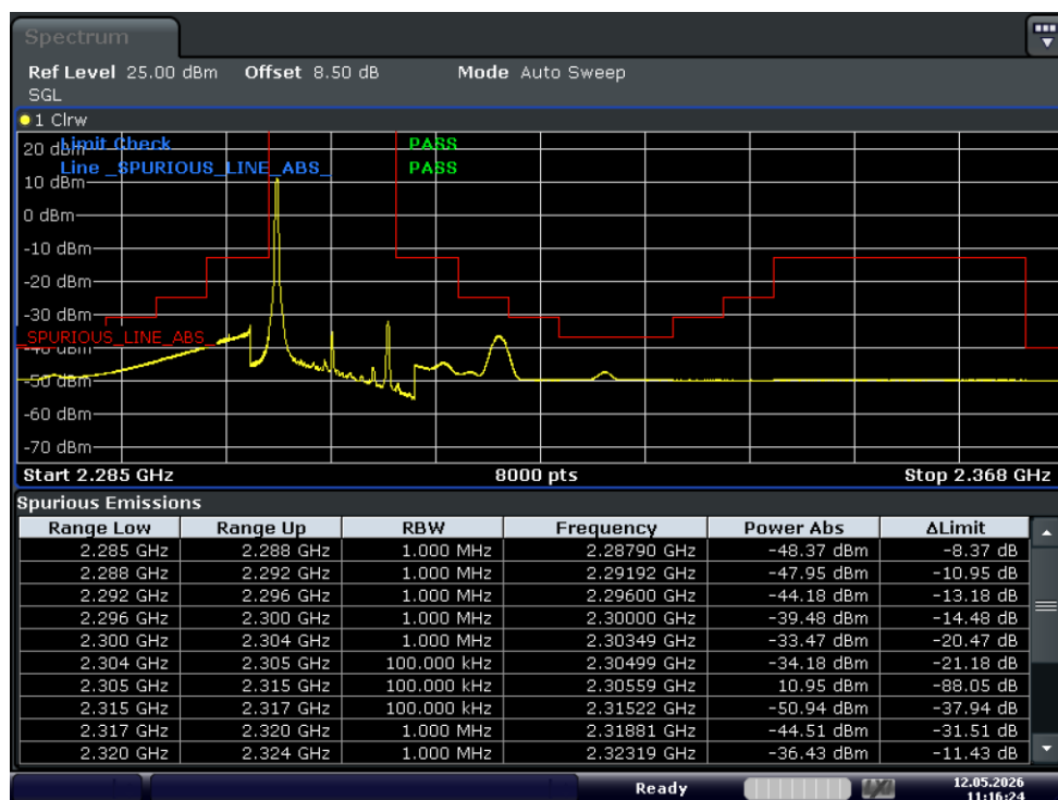
Test_Graph_band40(2305-2315)_2310MHz_10M_16QAM_1RB#LOW_Band edge
