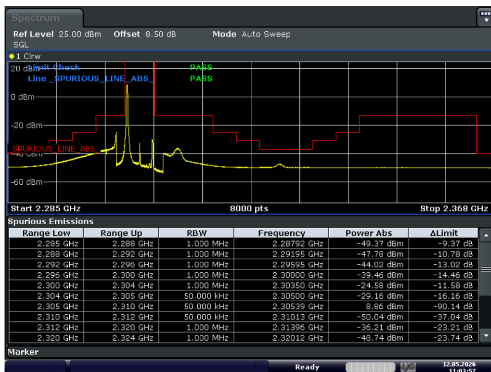
Test_Graph_band40(2305-2315)_2307.5MHz_5M_QPSK_1RB#LOW_Band edge
