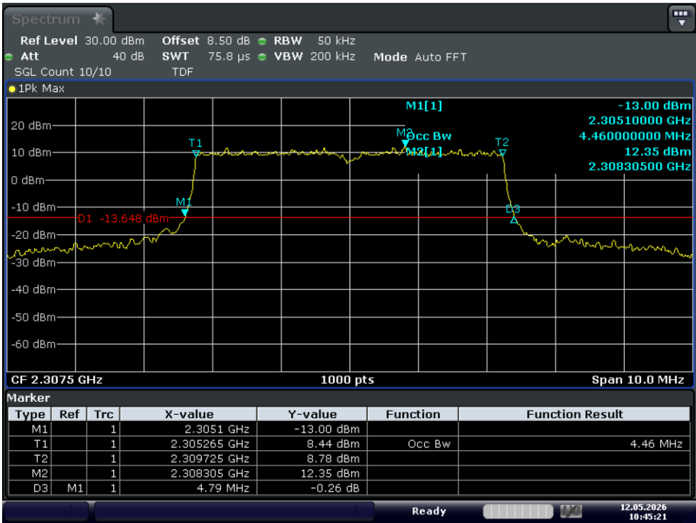
Test_Graph_band40(2305-2315)_2307.5MHz_5M_16QAM_25RB#LOW_OBW&EBW
