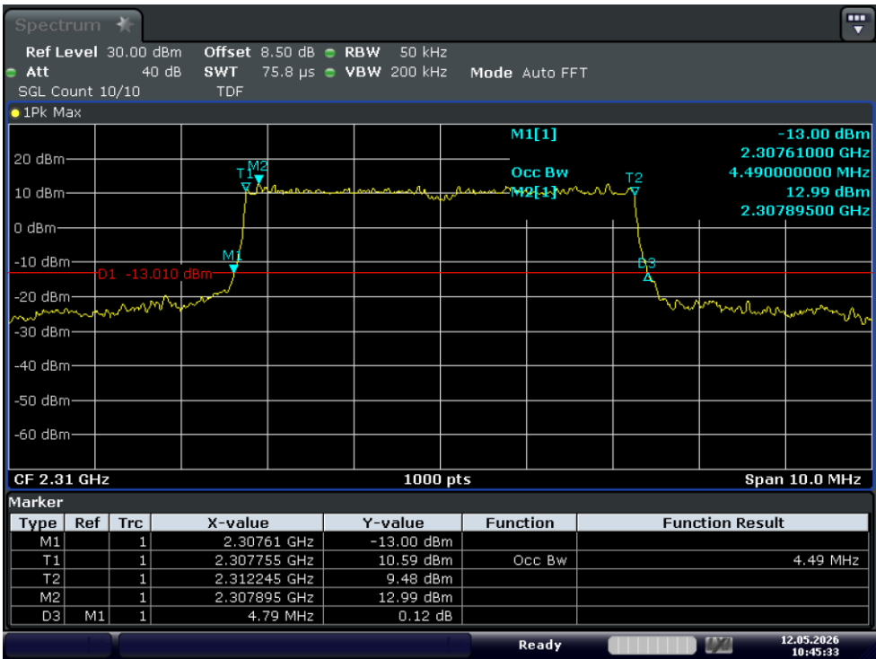
Test_Graph_band40(2305-2315)_2310MHz_5M_16QAM_25RB#LOW_OBW&EBW
