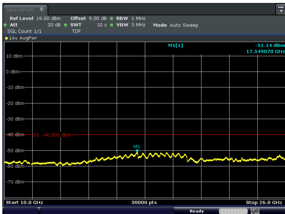
Test_Graph_band40(2305-2315)_2307.5MHz_5M_QPSK_25RB#LOW_10G_26.0G_TX
