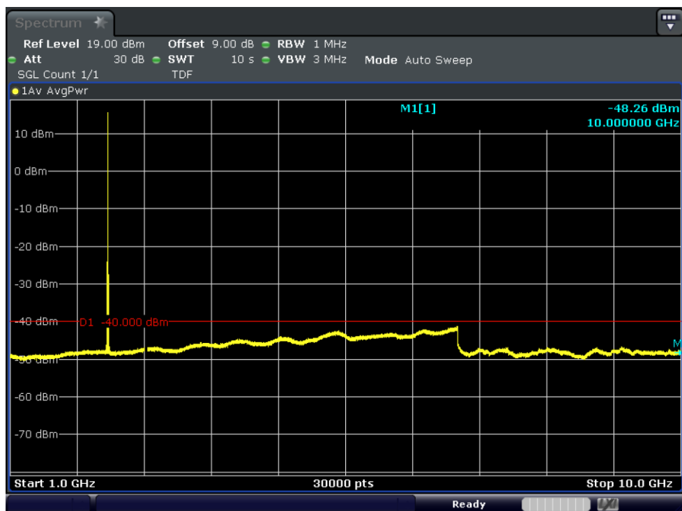
Test_Graph_band40(2305-2315)_2310MHz_5M_QPSK_25RB#LOW_1G_10G_TX
