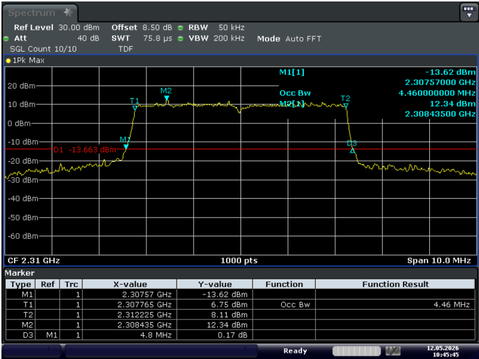
Test_Graph_band40(2305-2315)_2310MHz_5M_16QAM_25RB#LOW_OBW&EBW
