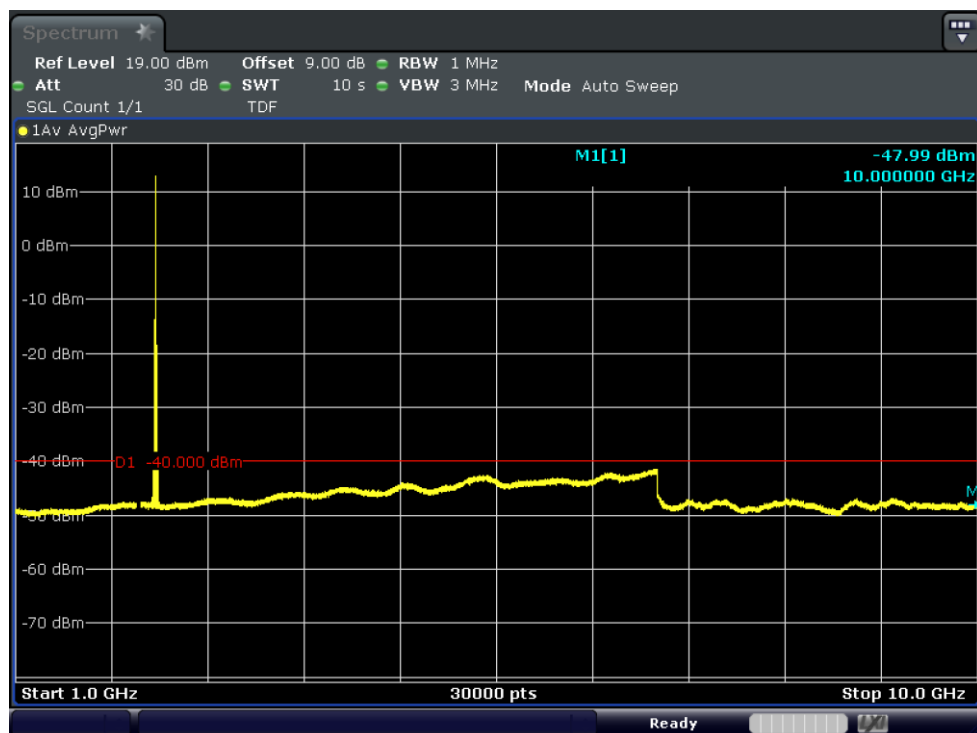
Test_Graph_band40(2305- 2315)_2310MHz_10M_QPSK_50RB#LOW_1G_10G_TX
