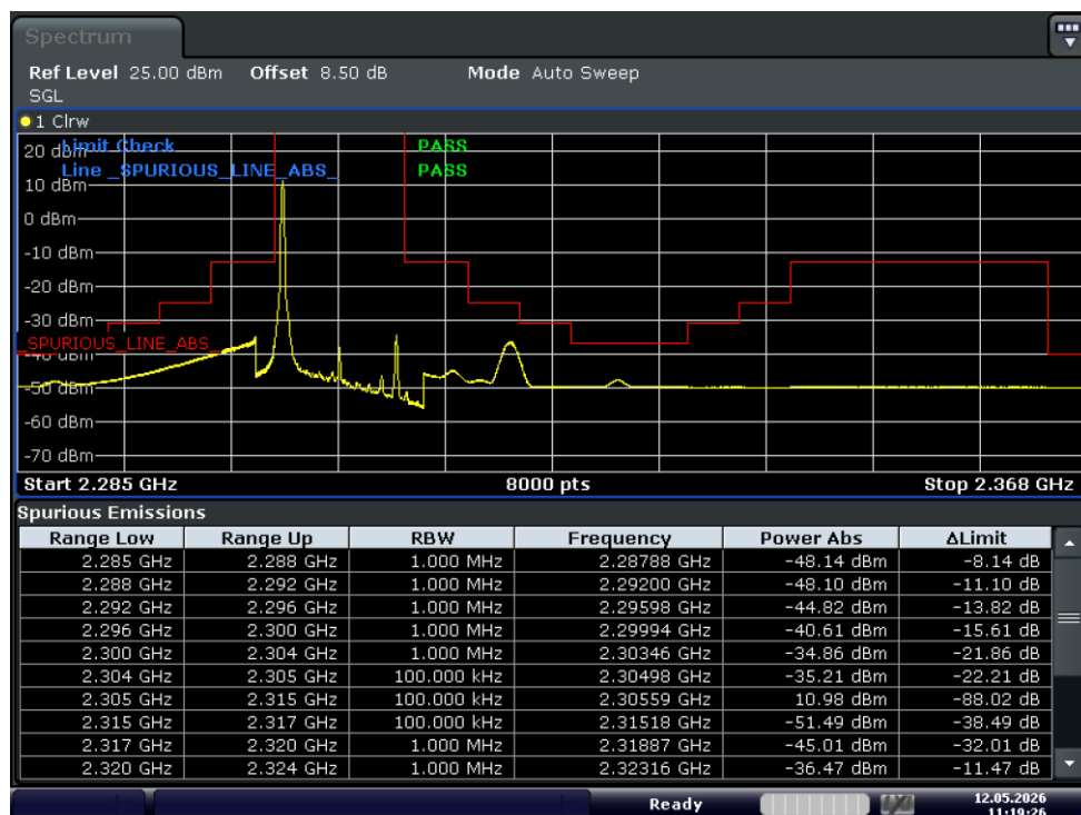
Test_Graph_band40(2305-2315)_2310MHz_10M_16QAM_1RB#LOW_Band edge
