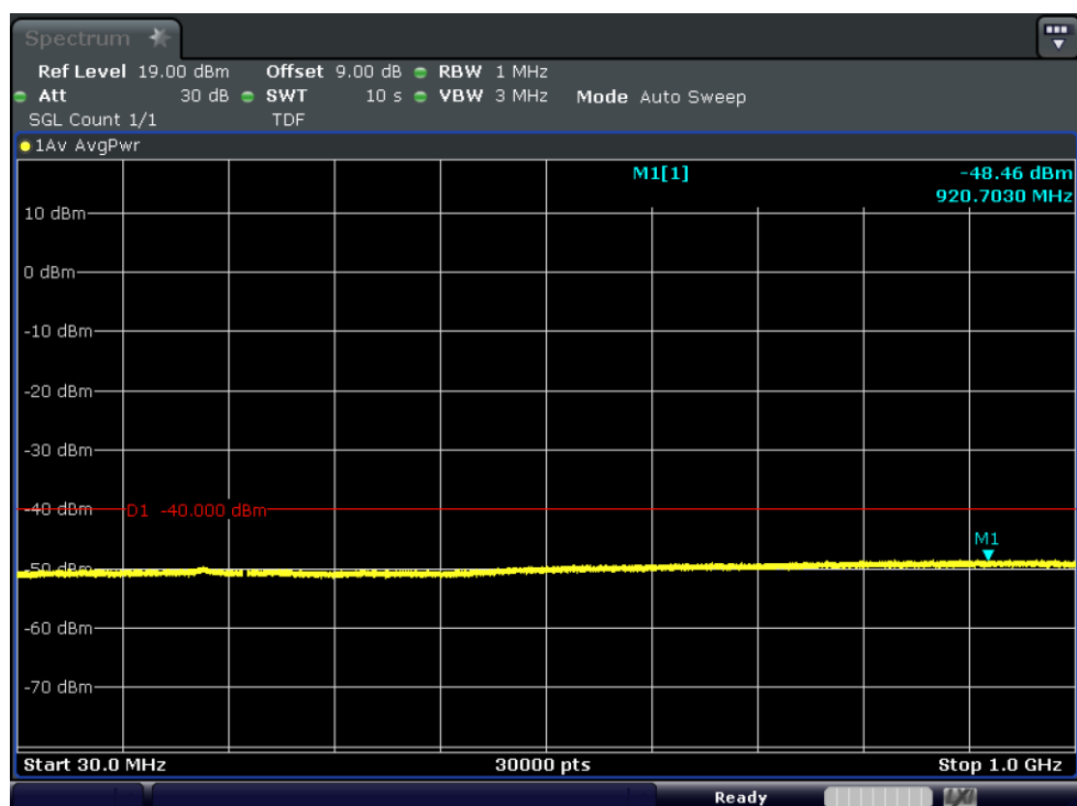
Test_Graph_band40(2305-2315)_2312.5MHz_5M_QPSK_25RB#LOW_30M_1G_TX
