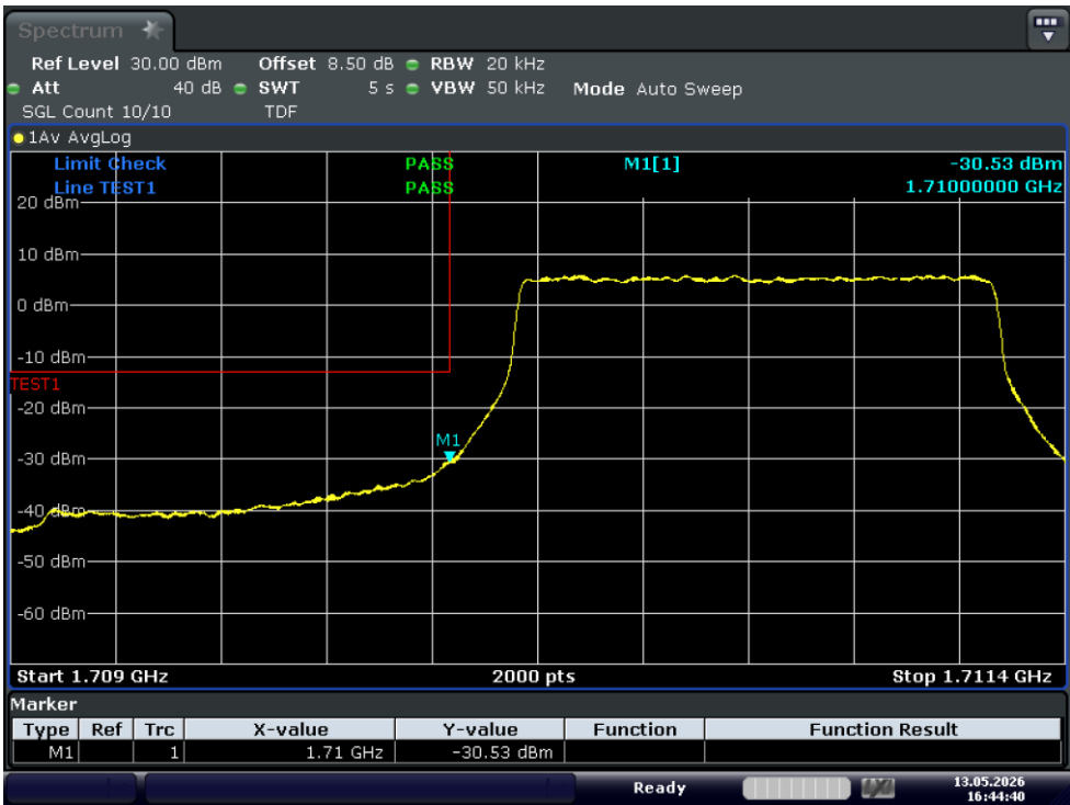
Test_Graph_band66_1710.7MHz_1.4M_QPSK_1RB#LOW_Band edge
