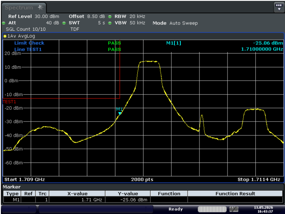
Test_Graph_band66_1710.7MHz_1.4M_QPSK_1RB#LOW_Band edge
