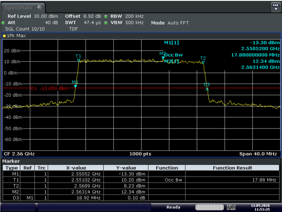
Test_Graph_band7_2560MHz_20M_QPSK_100RB#LOW_OBW&EBW
