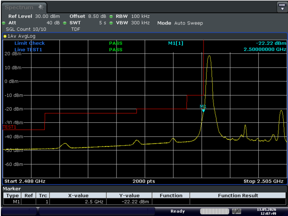
Test_Graph_band7_2502.5MHz_5M_16QAM_1RB#LOW_Band edge
