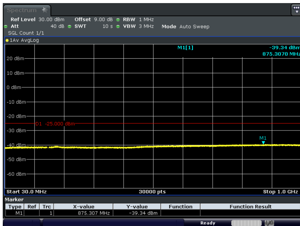
Test_Graph_band7_2502.5MHz_5M_QPSK_25RB#LOW_30M_1G_TX
