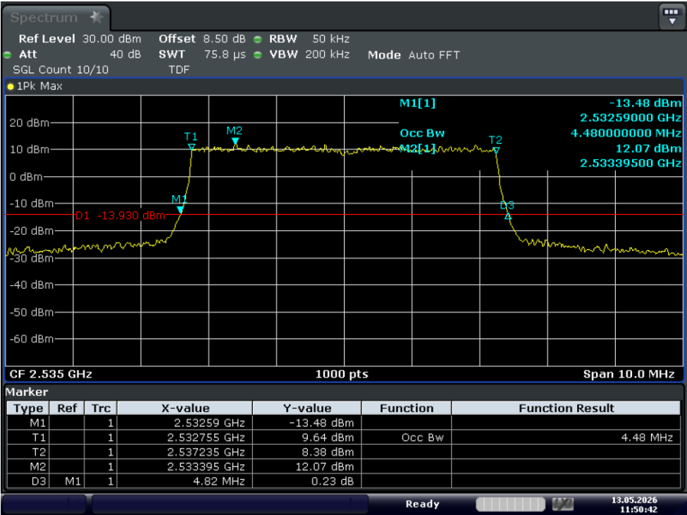
Test_Graph_band7_2535MHz_5M_16QAM_25RB#LOW_OBW&EBW
