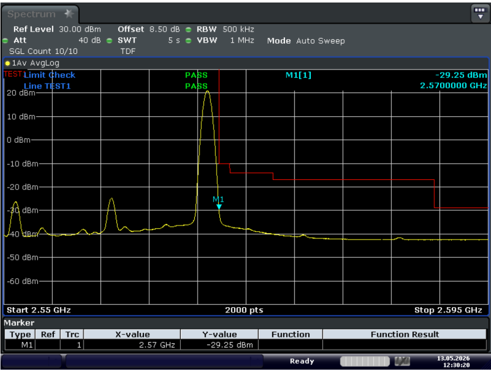
Test_Graph_band7_2560MHz_20M_QPSK_100RB#LOW_Band edge
