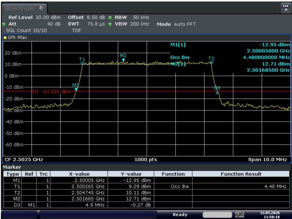
Test_Graph_band7_2502.5MHz_5M_16QAM_25RB#LOW_OBW&EBW
