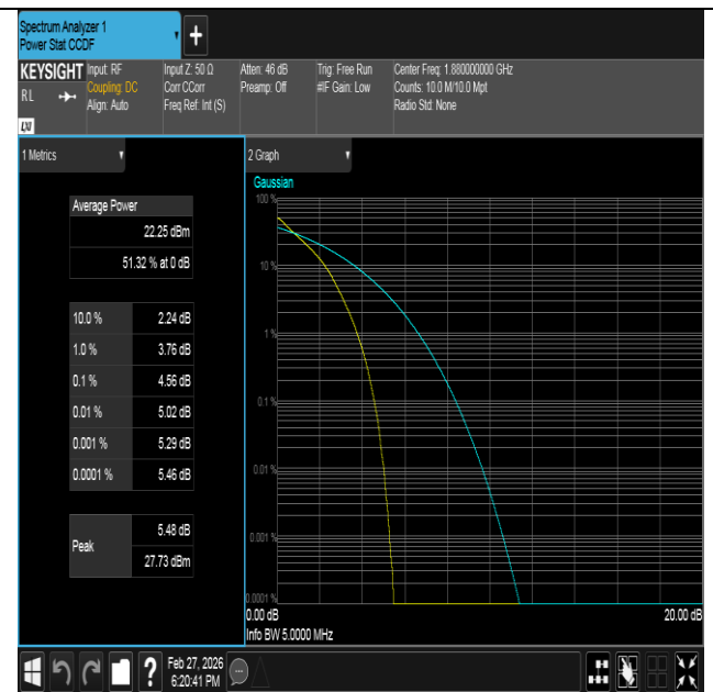
Band2-5MHz-QPSK-18900-25RB#0-PASS
