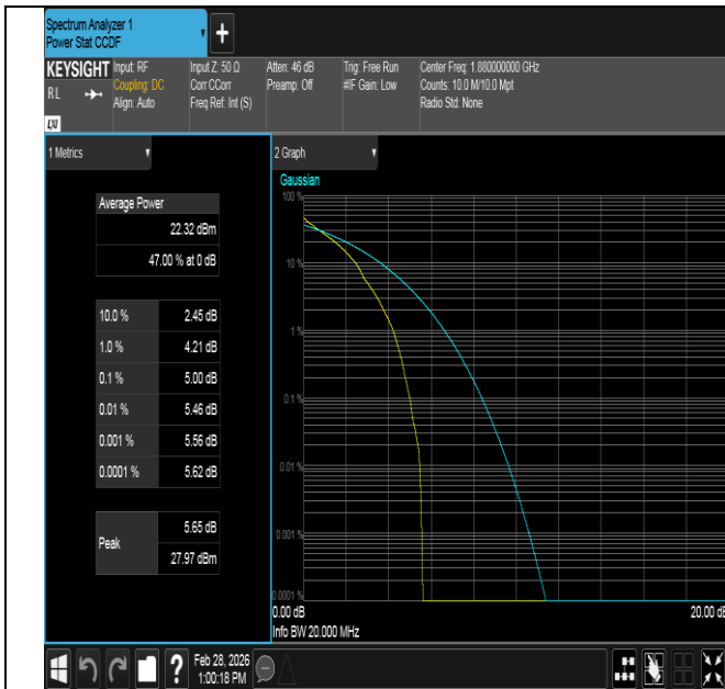
Band2-20MHz-QPSK-18900-1RB#0-PASS
