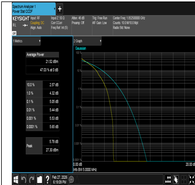
Band2-5MHz-QPSK-18625-1RB#0-PASS
