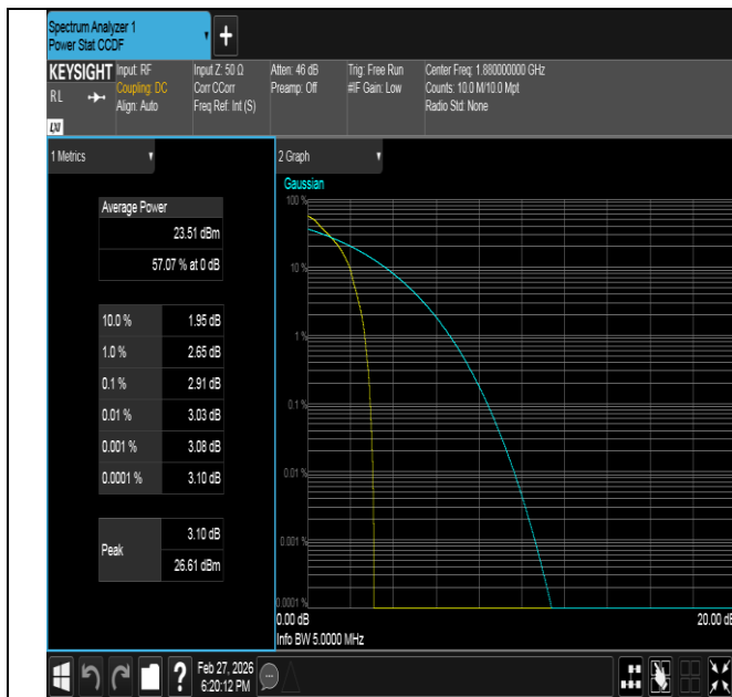
Band2-5MHz-QPSK-18900-1RB#0-PASS
