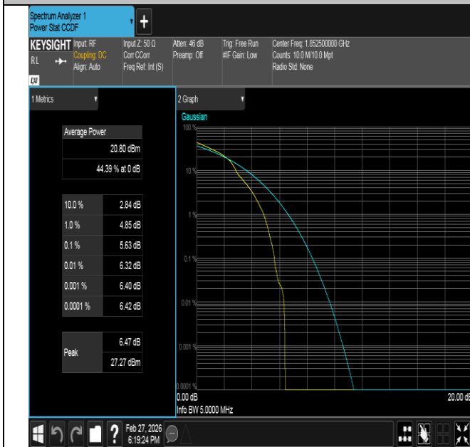
Band2-5MHz-16QAM-18625-1RB#0-PASS
