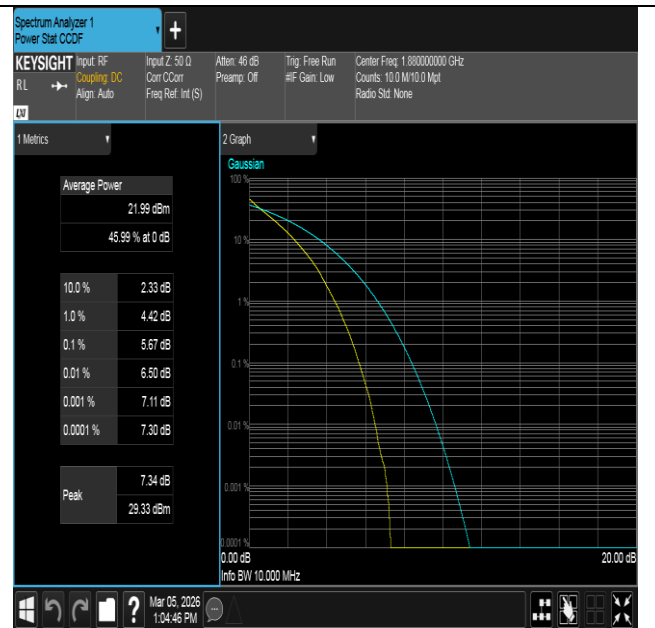
Band2-10MHz-QPSK-18900-50RB#0-PASS
