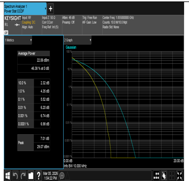
Band2-10MHz-QPSK-18650-50RB#0-PASS
