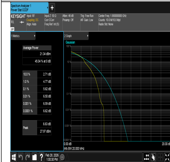
Band2-20MHz-16QAM-18900-1RB#0-PASS
