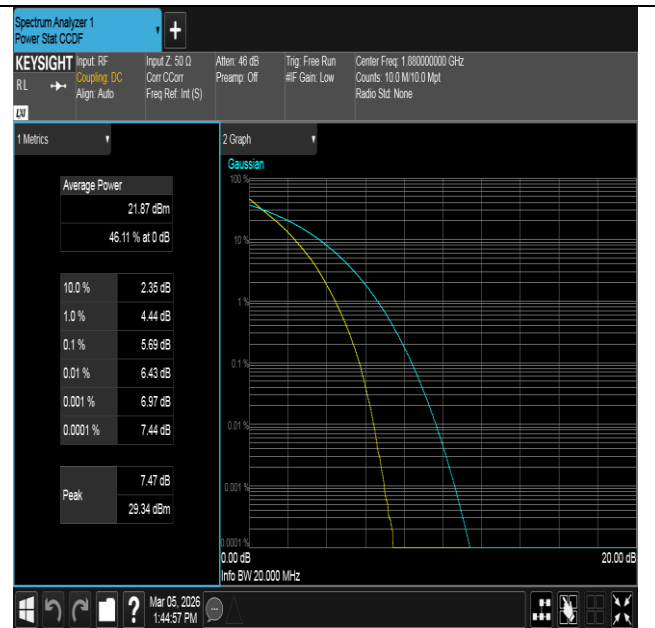
Band2-20MHz-QPSK-18900-100RB#0-PASS
