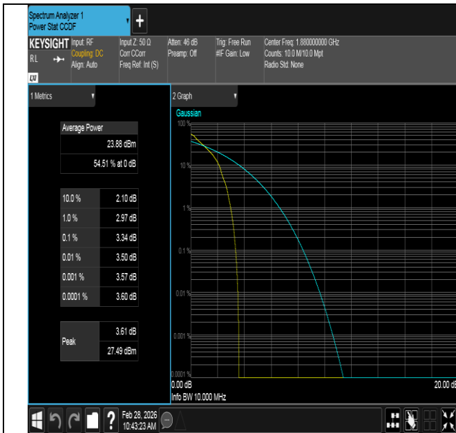
Band2-10MHz-QPSK-18900-1RB#0-PASS
