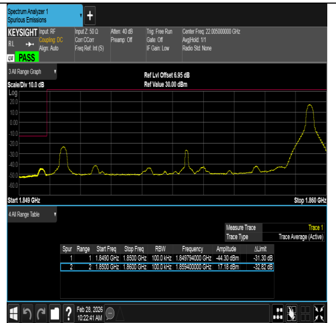
Band2-10MHz-QPSK-18650-1RB#49-PASS
