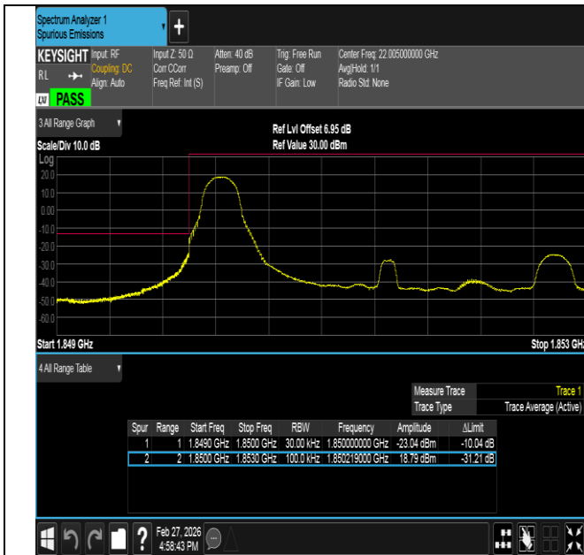
Band2-3MHz-QPSK-18615-1RB#0-PASS
