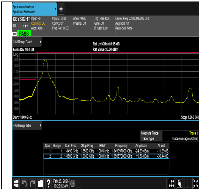
Band2-10MHz-QPSK-18650-1RB#0-PASS
