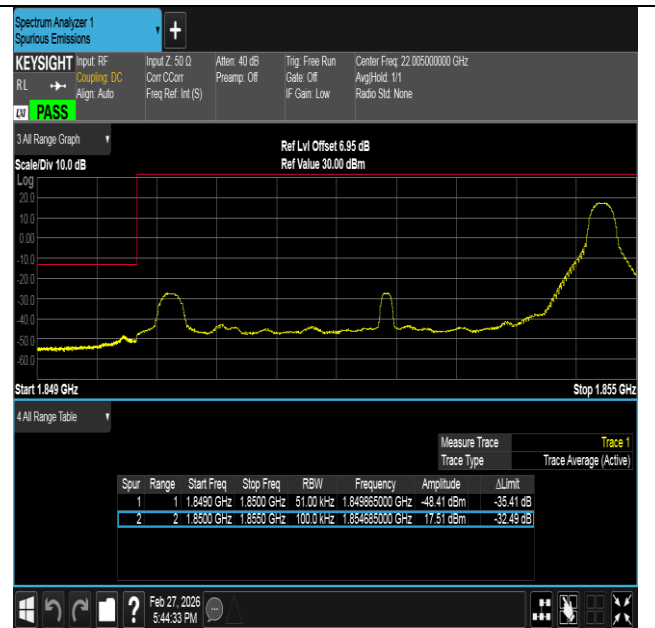
Band2-5MHz-QPSK-18625-1RB#24-PASS
