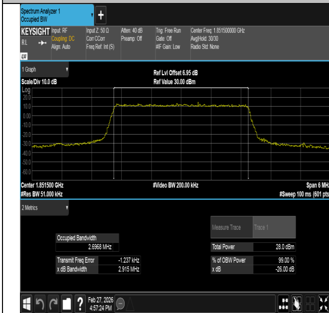
Band2-3MHz-QPSK-18615-15RB#0-PASS
