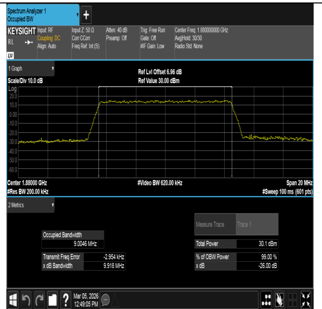
Band2-10MHz-16QAM-18900-50RB#0-PASS
