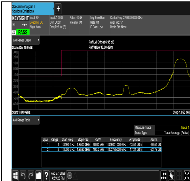
Band2-3MHz-16QAM-18615-1RB#14-PASS
