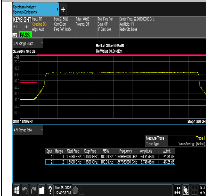
Band2-10MHz-QPSK-18650-50RB#0-PASS
