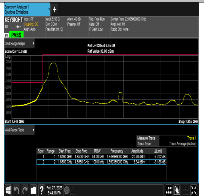
Band2-5MHz-16QAM-18625-1RB#0-PASS
