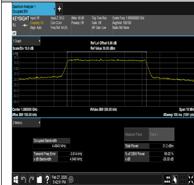
Band2-5MHz-QPSK-18900-25RB#0-PASS
