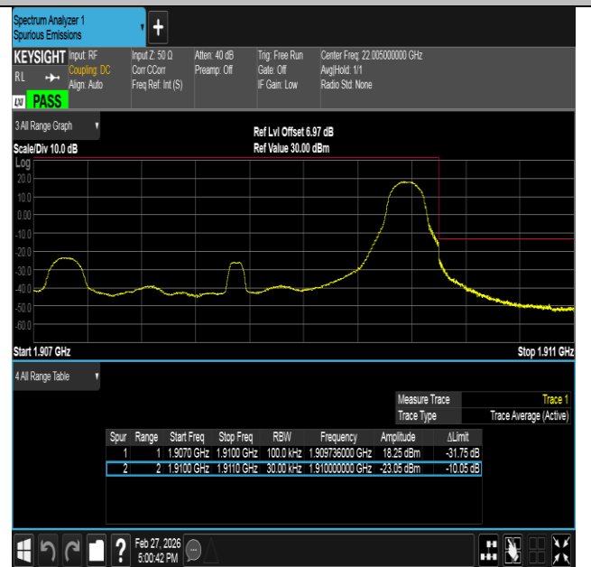
Band2-3MHz-QPSK-19185-1RB#14-PASS
