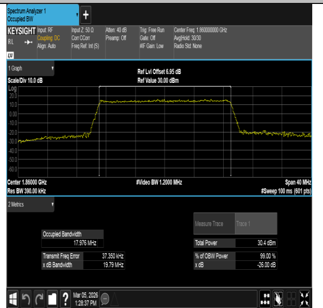
Band2-20MHz-16QAM-18700-100RB#0-PASS
