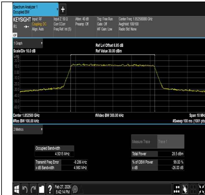
Band2-5MHz-QPSK-18625-25RB#0-PASS
