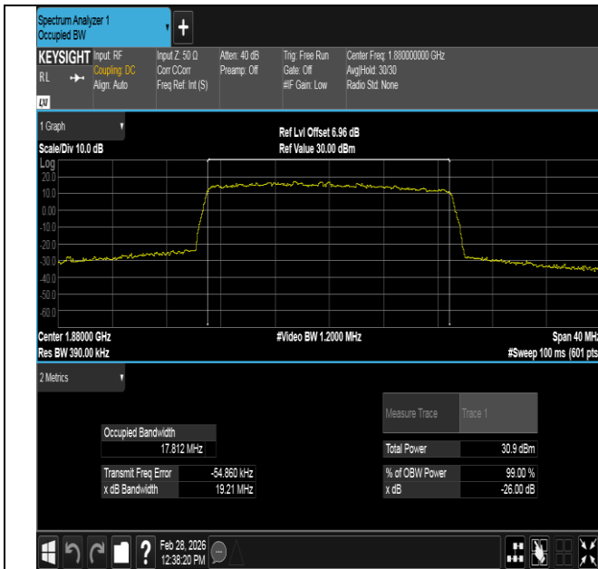
Band2-20MHz-QPSK-18900-100RB#0-PASS
