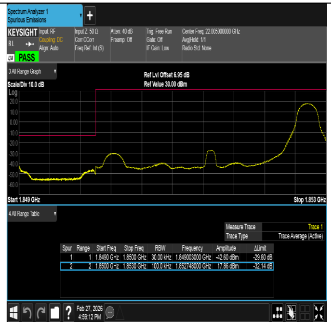
Band2-3MHz-QPSK-18615-1RB#14-PASS
