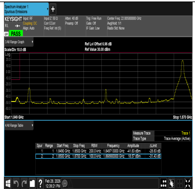
Band2-20MHz-QPSK-18700-1RB#99-PASS
