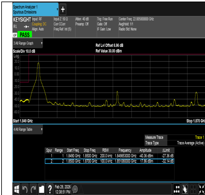
Band2-20MHz-QPSK-18700-1RB#0-PASS
