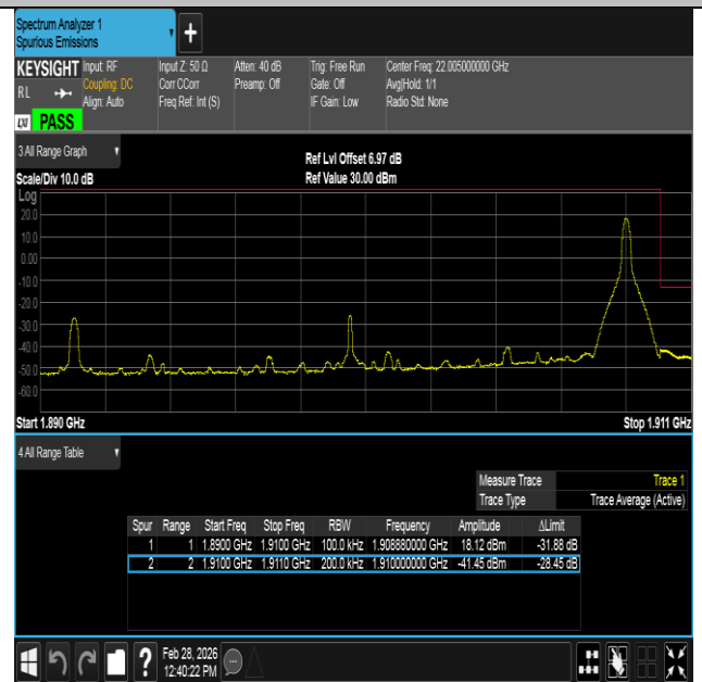
Band2-20MHz-QPSK-19100-1RB#99-PASS
