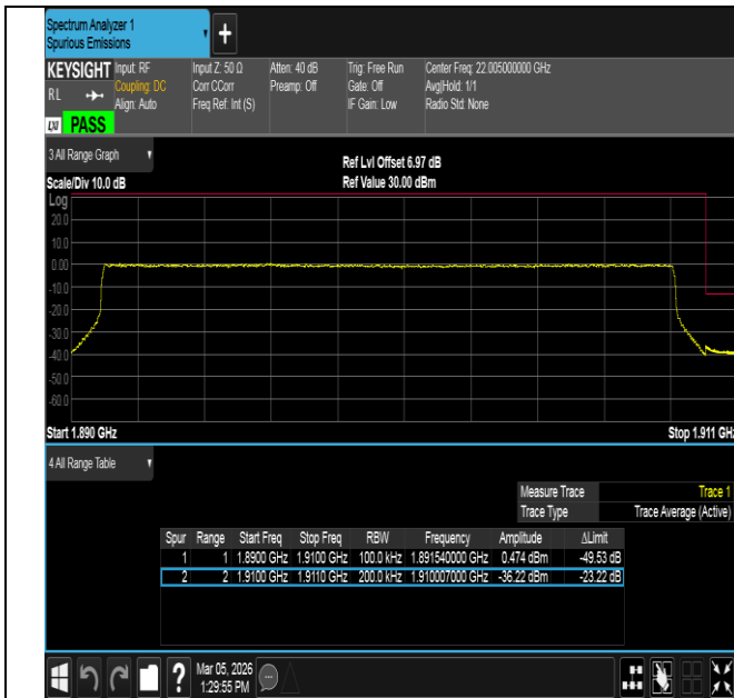
Band2-20MHz-QPSK-19100-100RB#0-PASS
