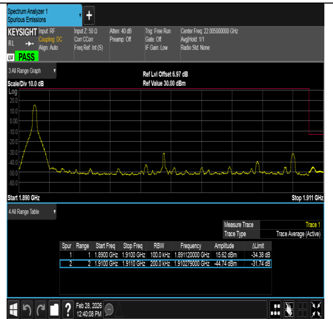
Band2-20MHz-16QAM-19100-1RB#0-PASS
