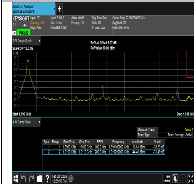
Band2-20MHz-QPSK-19100-1RB#0-PASS
