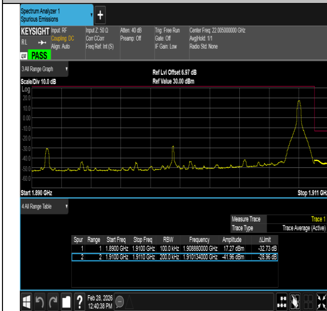
Band2-20MHz-16QAM-19100-1RB#99-PASS
