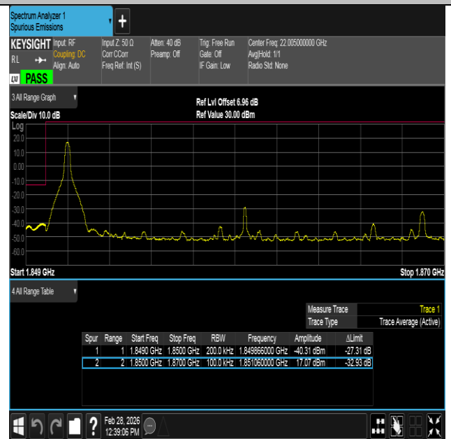
Band2-20MHz-16QAM-18700-1RB#0-PASS
