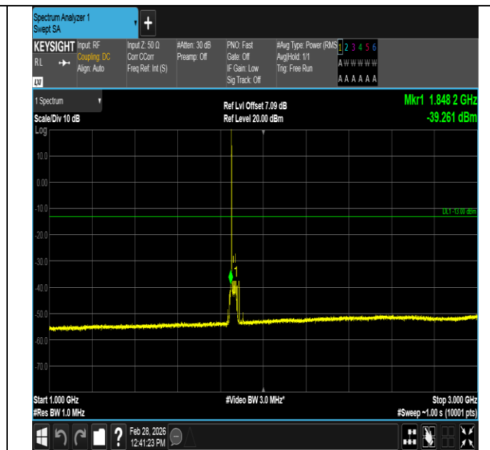
Band2-20MHz-QPSK-18700-1RB#0-1000~3000-PASS
