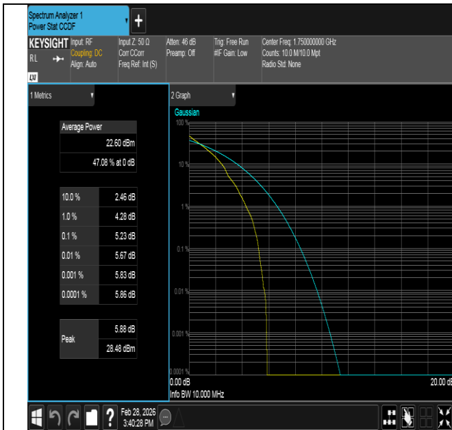
Band4-10MHz-QPSK-20350-1RB#0-PASS
