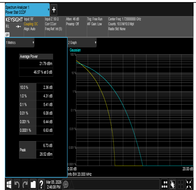
Band4-20MHz-QPSK-20050-100RB#0-PASS
