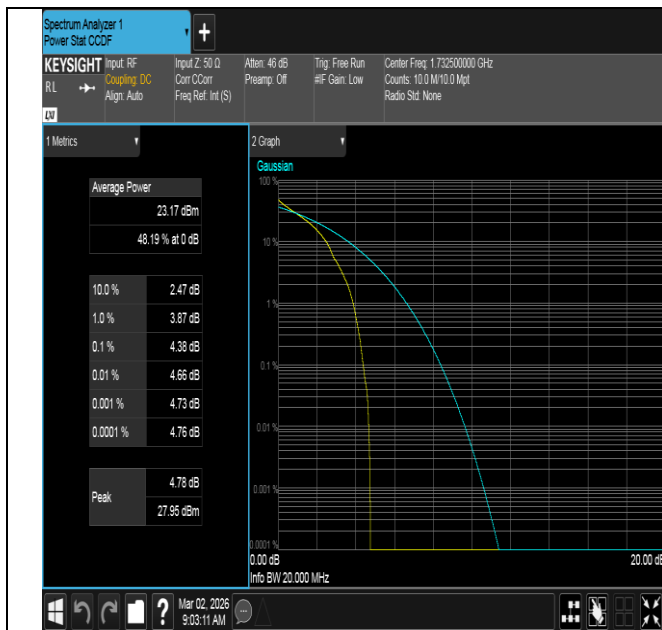
Band4-20MHz-QPSK-20175-1RB#0-PASS
