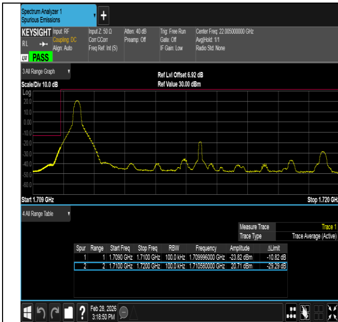
Band4-10MHz-QPSK-20000-1RB#0-PASS
