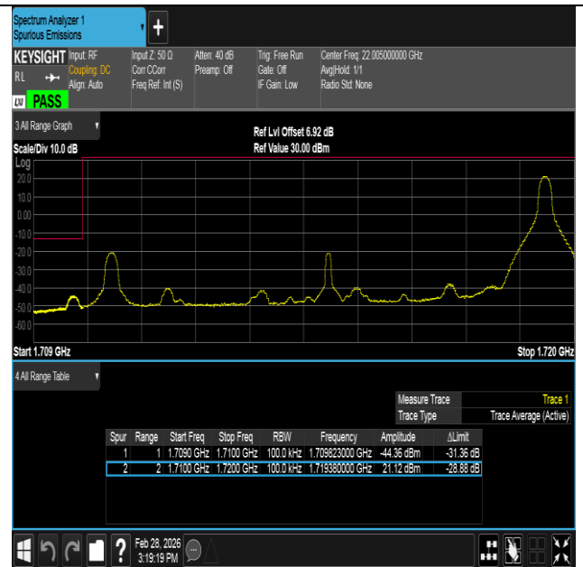
Band4-10MHz-QPSK-20000-1RB#49-PASS
