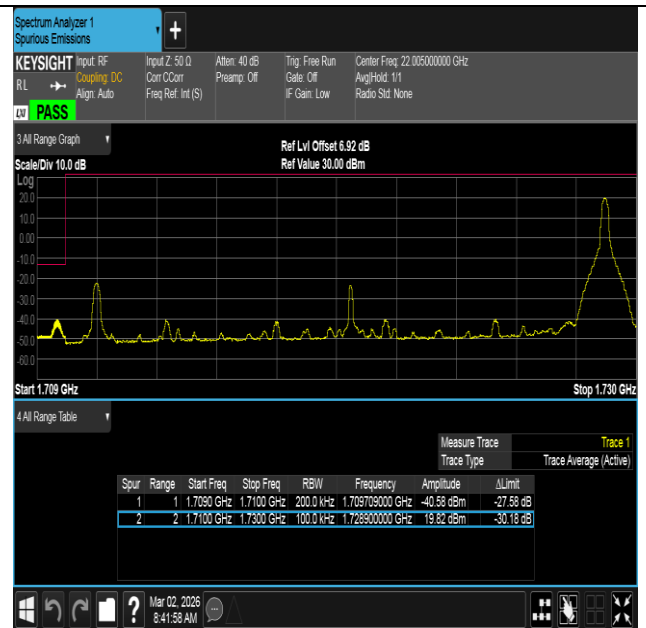
Band4-20MHz-QPSK-20050-1RB#99-PASS
