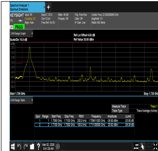
Band4-20MHz-QPSK-20050-1RB#0-PASS
