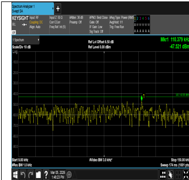
Band4-10MHz-QPSK-20000-50RB#0-0.009~0.15-PASS
