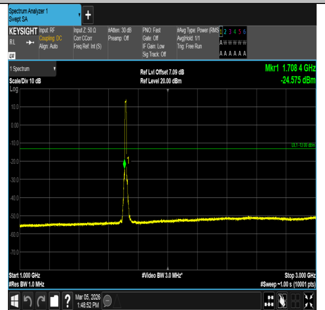
Band4-10MHz-QPSK-20000-50RB#0-1000~3000-PASS
