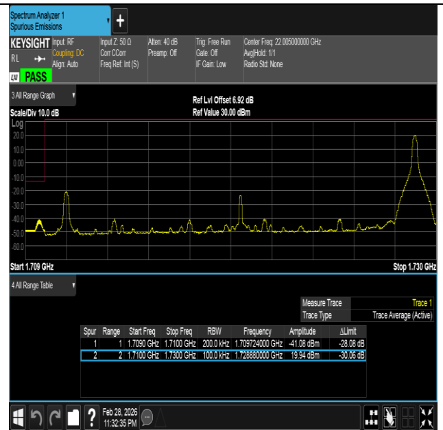
Band66-20MHz-QPSK-132072-1RB#99-PASS
