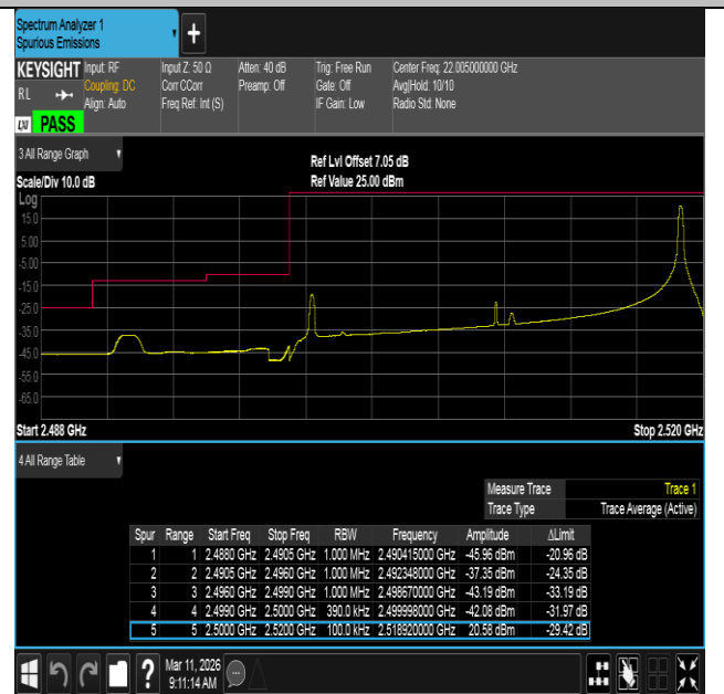
Band7-20MHz-QPSK-20850-1RB#99-PASS
