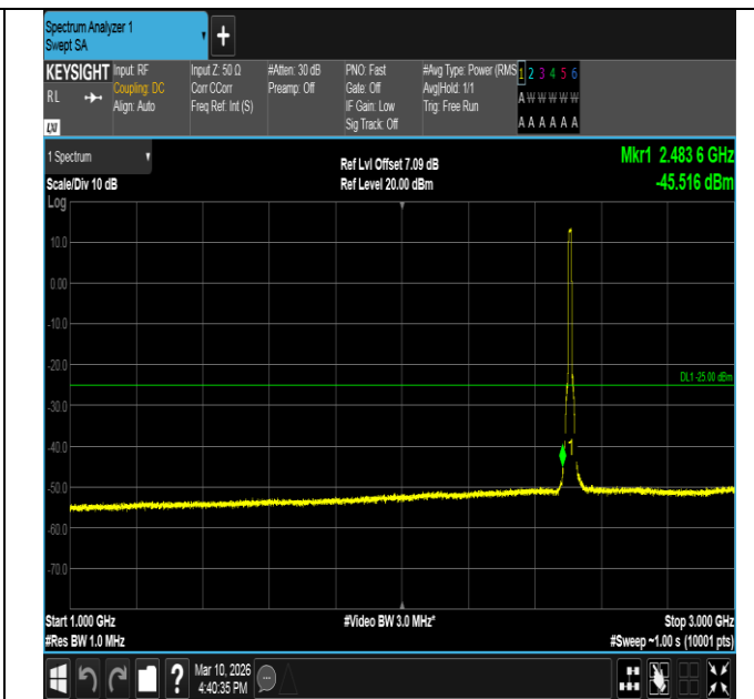
Band7-10MHz-QPSK-20800-50RB#0-1000~3000-PASS
