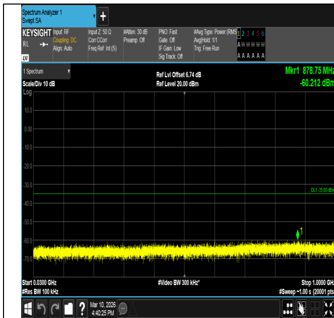
Band7-10MHz-QPSK-20800-50RB#0-30~1000-PASS
