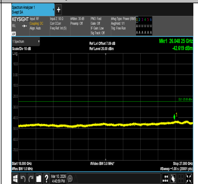
Band7-10MHz-QPSK-20800-50RB#0-18000~27000-PASS
