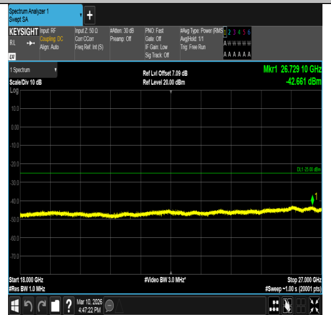
Band7-10MHz-QPSK-21100-50RB#0-18000~27000-PASS
