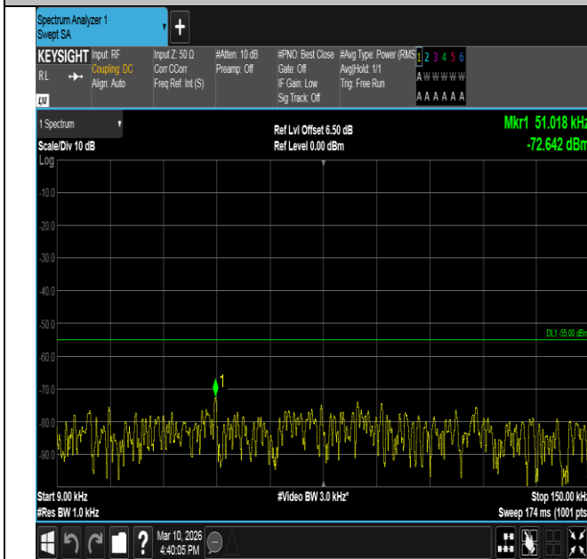
Band7-10MHz-QPSK-20800-50RB#0-0.009~0.15-PASS
