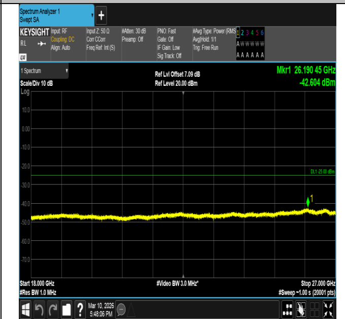
Band7-15MHz-16QAM-20825-1RB#74-18000~27000-PASS
