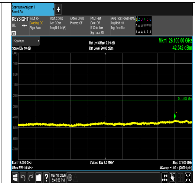
Band7-15MHz-16QAM-20825-1RB#0-18000~27000-PASS
