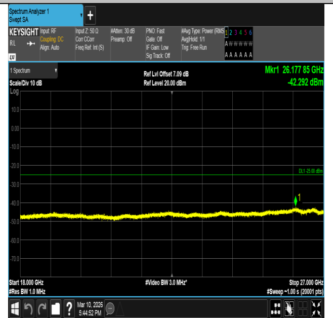
Band7-15MHz-QPSK-20825-1RB#0-18000~27000-PASS
