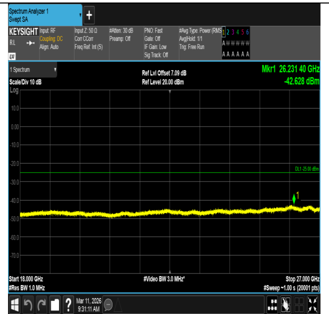
Band7-20MHz-QPSK-20850-1RB#99-18000~27000-PASS
