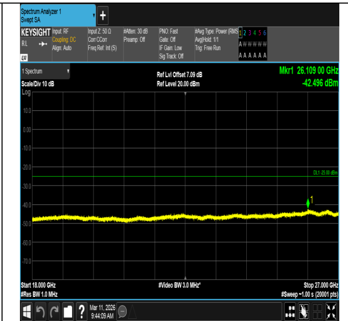
Band7-20MHz-QPSK-21350-1RB#99-18000~27000-PASS
