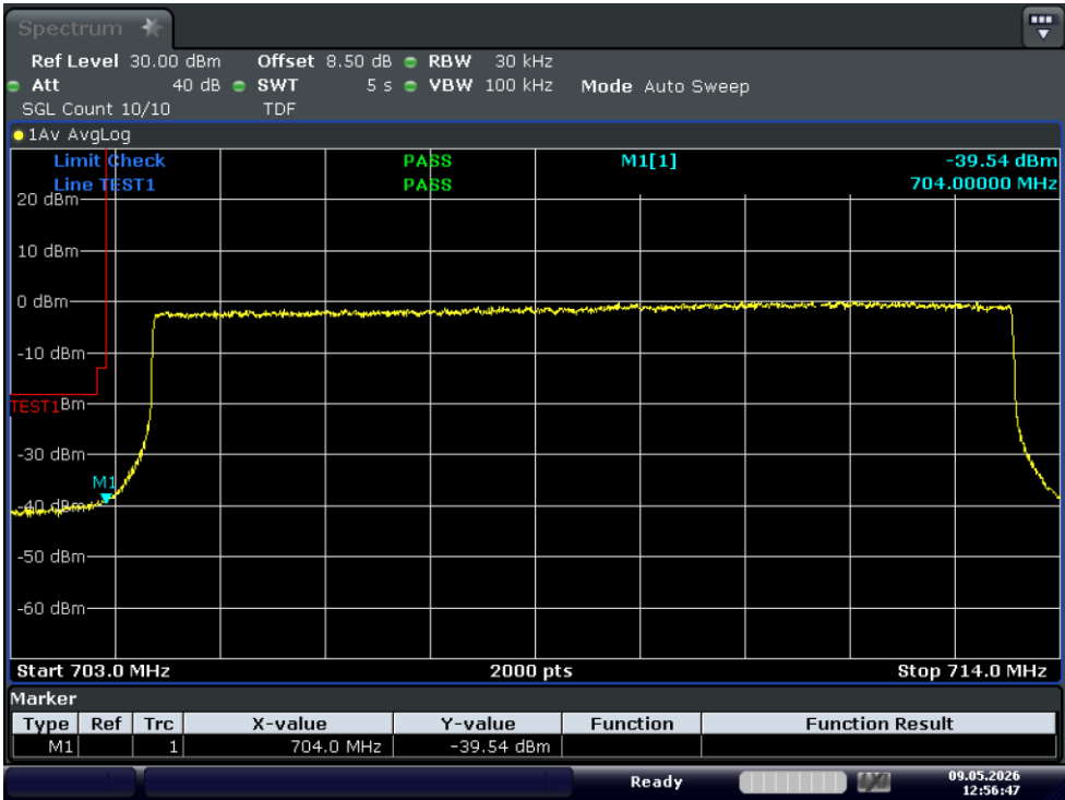
Test_Graph_band17_709MHz_10M_QPSK_50RB#LOW_Band edge
