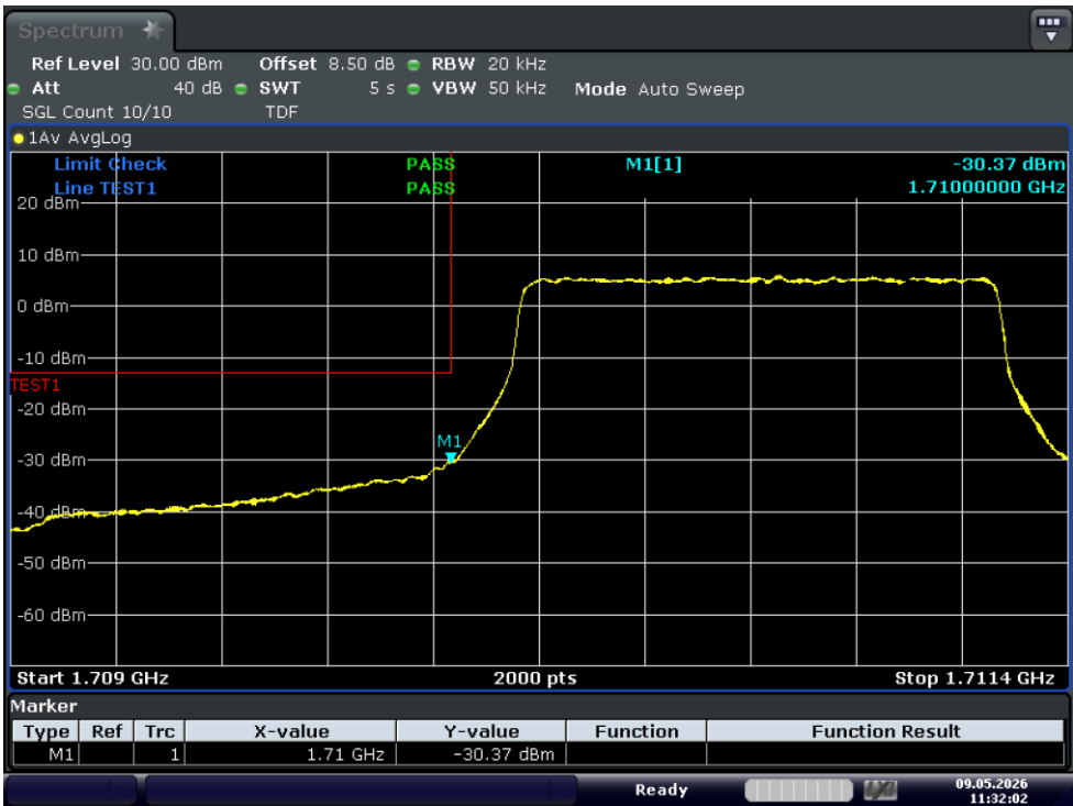
Test_Graph_band66_1710.7MHz_1.4M_16QAM_1RB#LOW_Band edge
