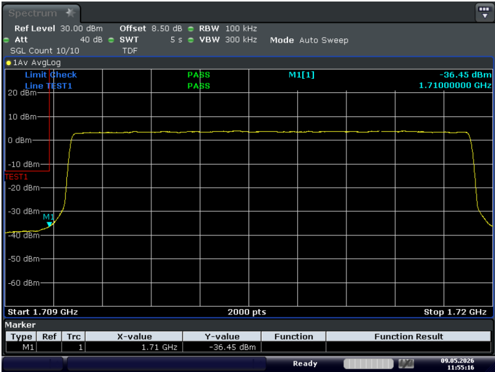
Test_Graph_band66_1715MHz_10M_QPSK_50RB#LOW_Band edge
