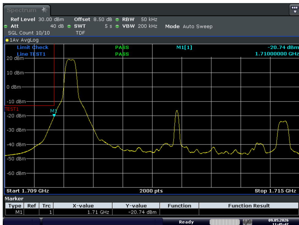
Test_Graph_band66_1712.5MHz_5M_QPSK_1RB#LOW_Band edge
