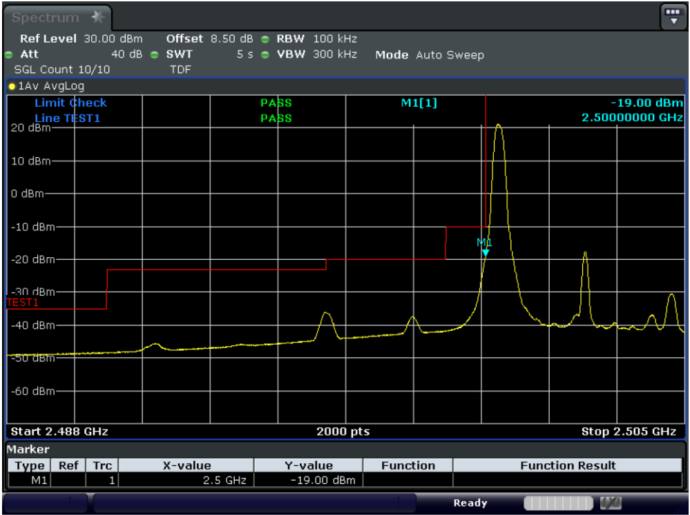
Test_Graph_band7_2502.5MHz_5M_QPSK_1RB#LOW_Band edge
