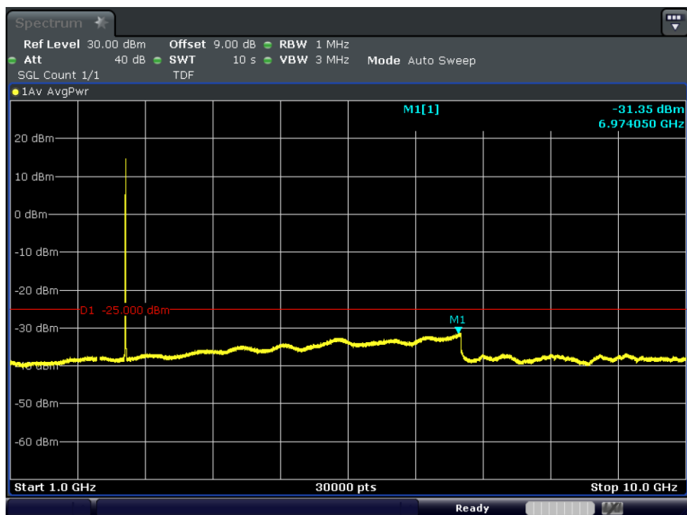
Test_Graph_band7_2535MHz_5M_QPSK_25RB#LOW_1G_10G_TX
