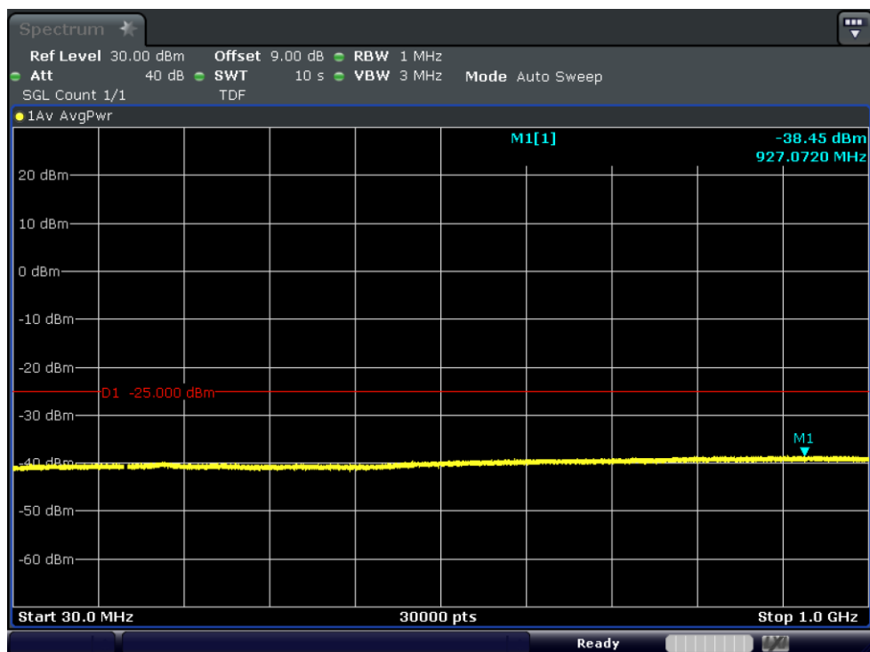
Test_Graph_band7_2507.5MHz_15M_QPSK_75RB#LOW_30M_1G_TX
