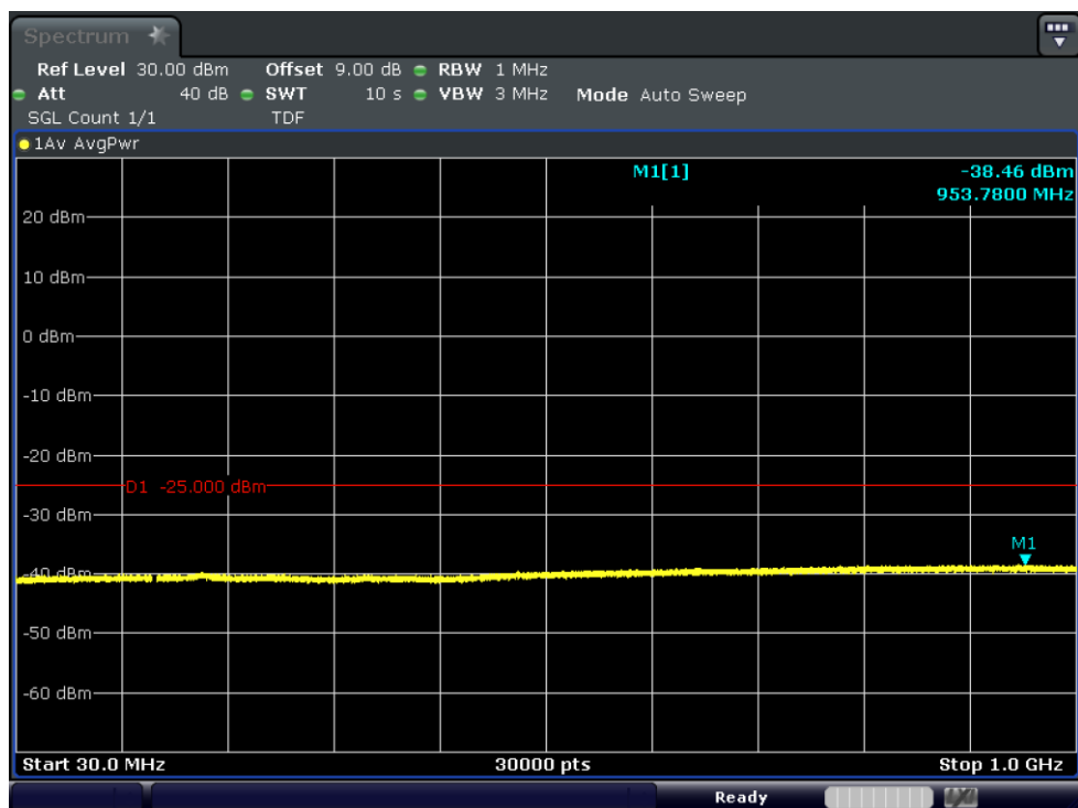
Test_Graph_band7_2567.5MHz_5M_QPSK_25RB#LOW_30M_1G_TX
