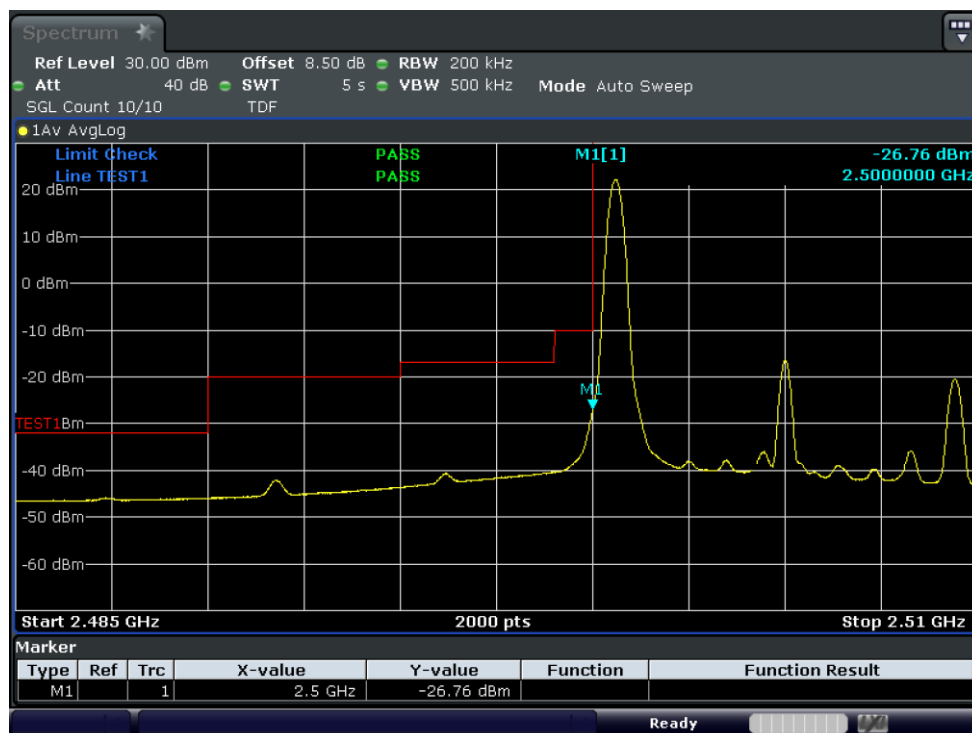
Test_Graph_band7_2505MHz_10M_16QAM_1RB#LOW_Band edge
