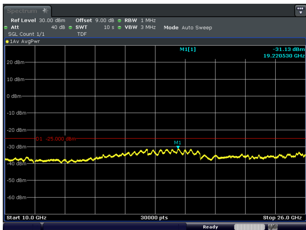
Test_Graph_band7_2535MHz_20M_QPSK_100RB#LOW_10G_26.0G_TX
