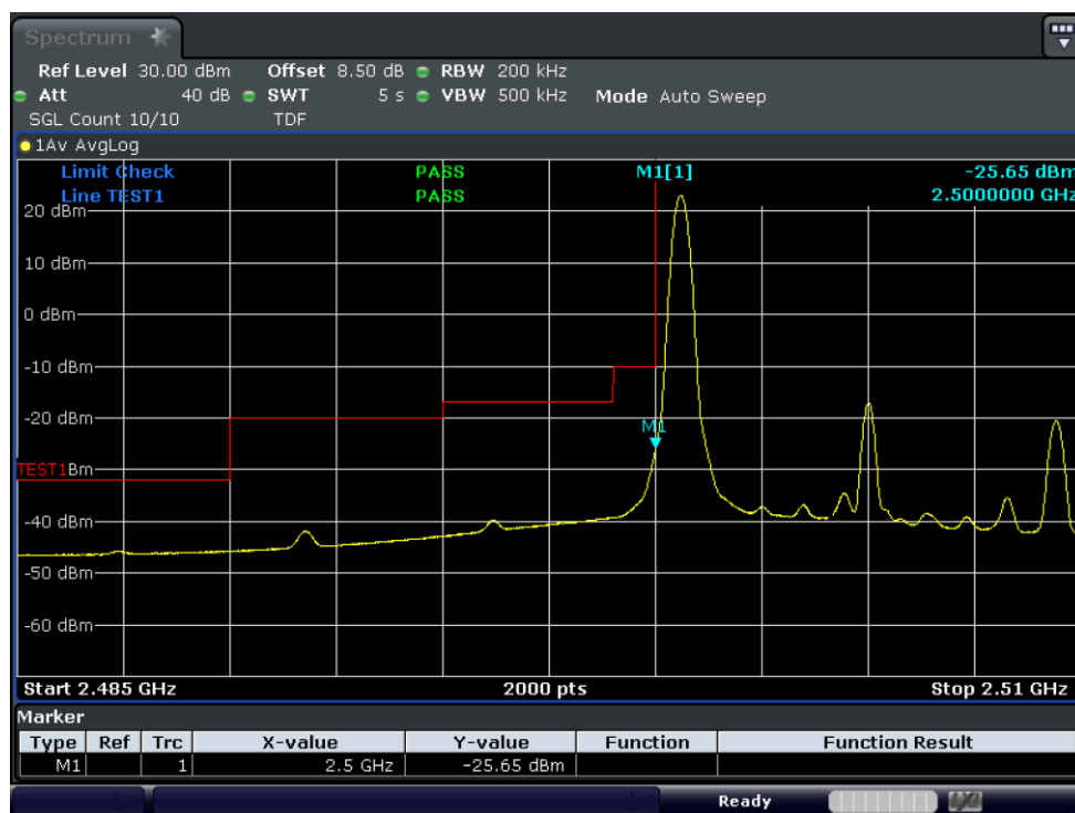
Test_Graph_band7_2505MHz_10M_16QAM_1RB#LOW_Band edge
