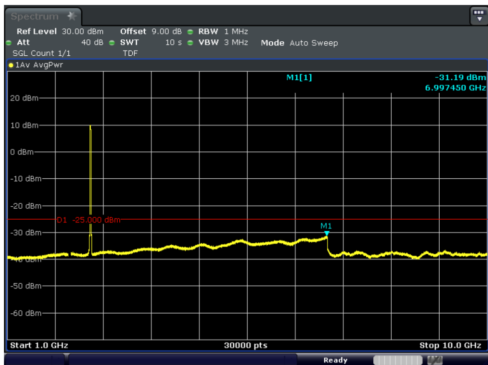
Test_Graph_band7_2560MHz_20M_QPSK_100RB#LOW_1G_10G_TX
