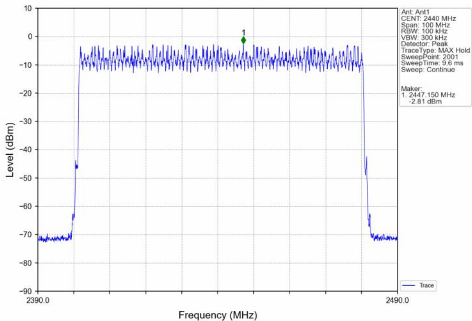
8DPSK_3DH5_HOPP_2440MHz_Ant1_NTNV
