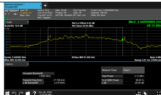
BLE 2M_Channel 19
