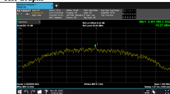
BLE 1M_Channel 0
