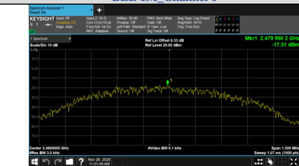
BLE 1M_Channel 39
