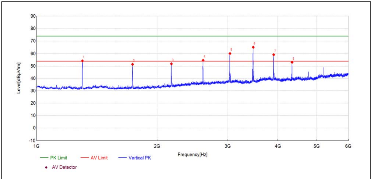
(Antenna Vertical, 1GHz to 6GHz)
