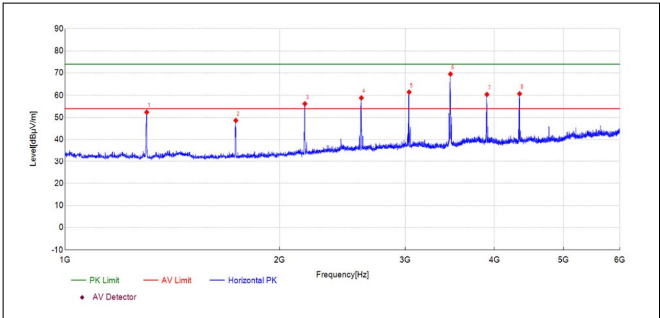
(Antenna Horizontal, 1GHz to 6GHz)
