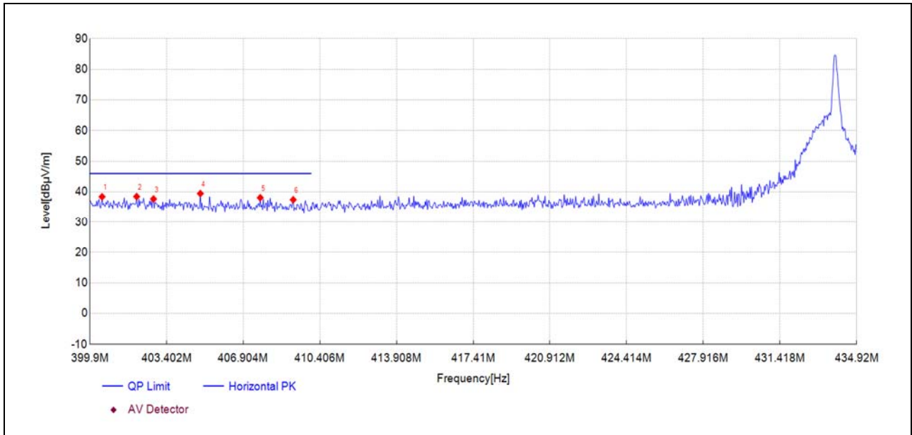
(Antenna Horizontal)
