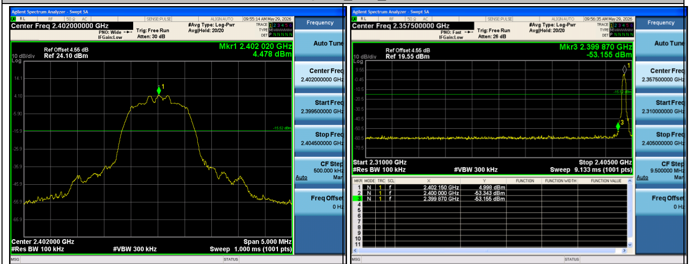
\pi/4 -DQPSK_Low_Hop_2402
