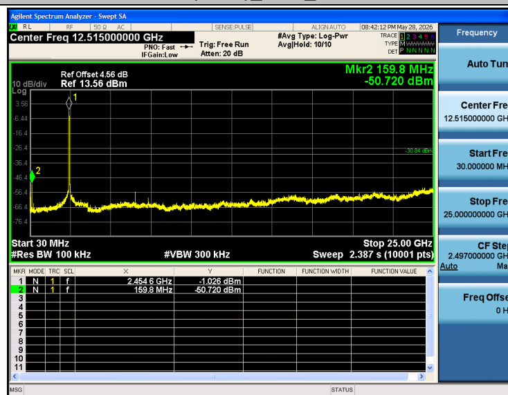
802.11n(HT40)_2462_30~25000
