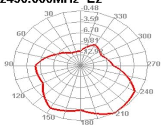
2450.000MHz E2
