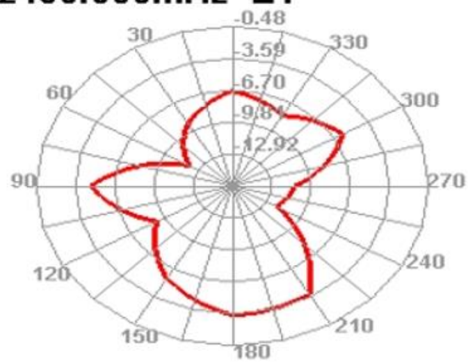
2450.000MHz E1
