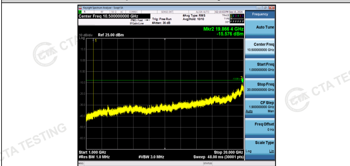
Band2-3MHz-QPSK-18900-1RB#0-Range2:1000~20000MHz
