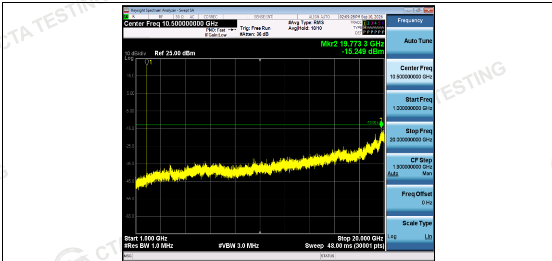
Band2-3MHz-16QAM-18615-1RB#0-Range2:1000~20000MHz
