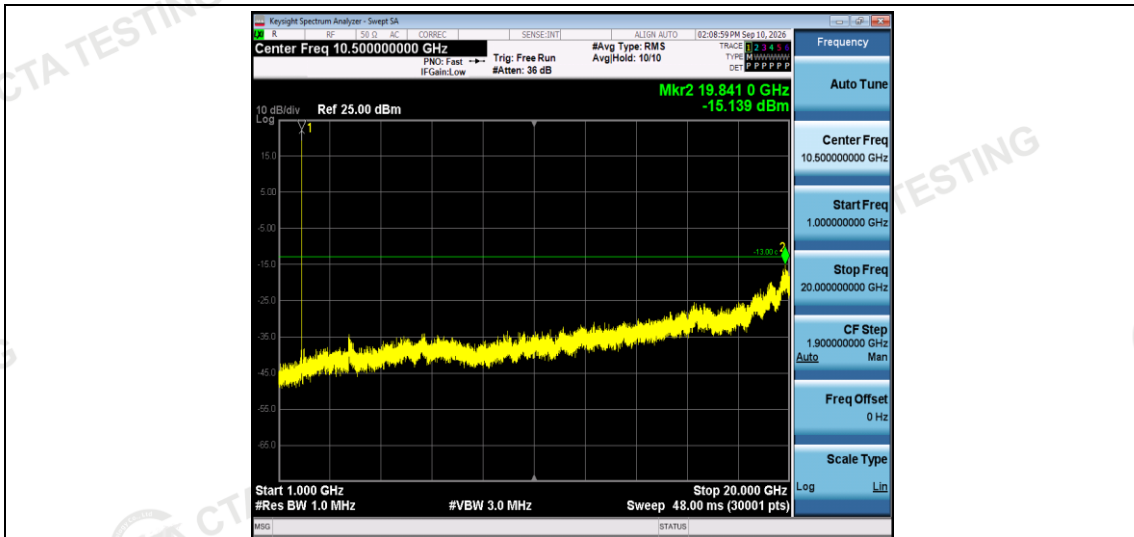
Band2-3MHz-QPSK-18615-1RB#0-Range2:1000~20000MHz
