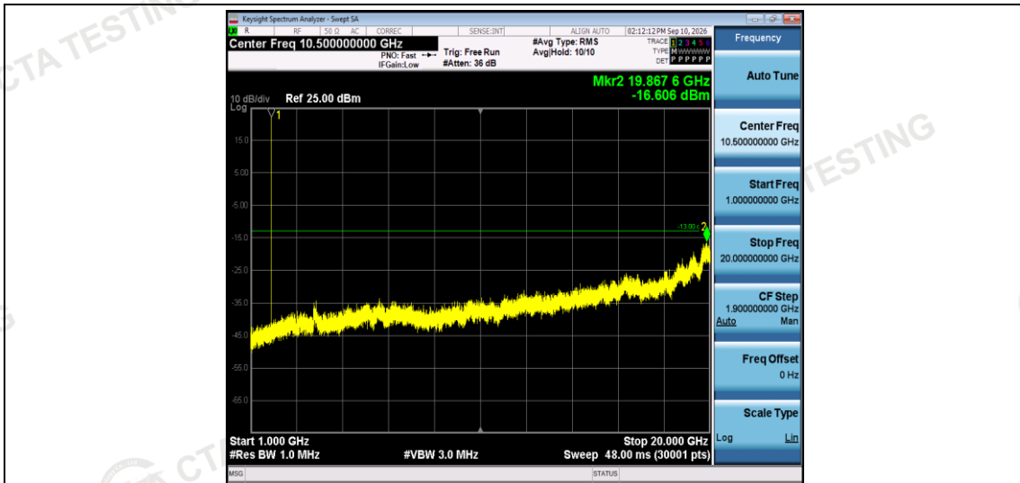
Band2-5MHz-QPSK-18625-1RB#0-Range2:1000~20000MHz
