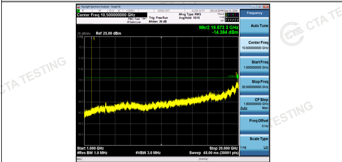
Band2-5MHz-QPSK-19175-1RB#0-Range2:1000~20000MHz
