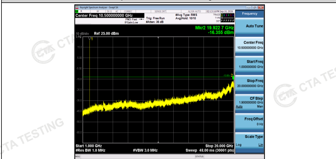
Band2-5MHz-QPSK-18900-1RB#0-Range2:1000~20000MHz
