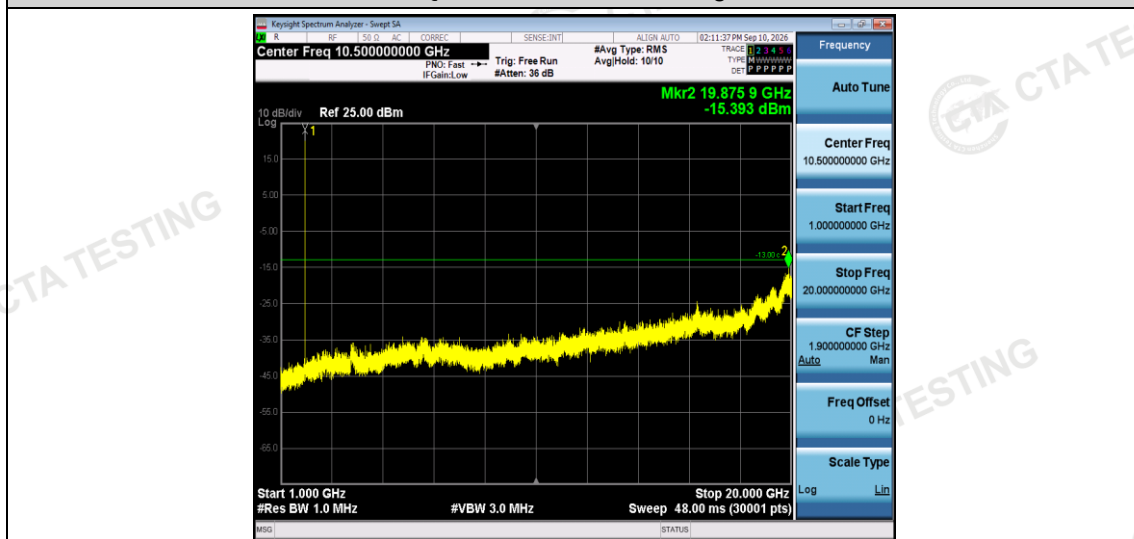
Band2-3MHz-16QAM-19185-1RB#0-Range2:1000~20000MHz
