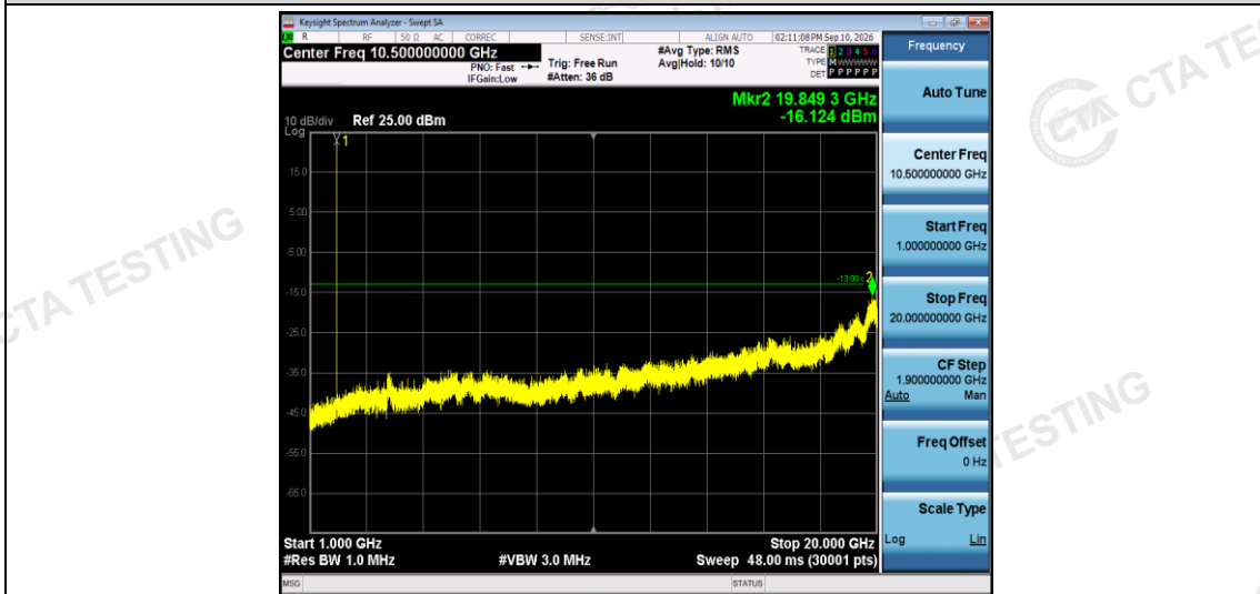
Band2-3MHz-QPSK-19185-1RB#0-Range2:1000~20000MHz
