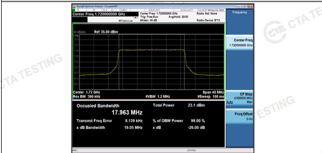
Band4-20MHz-QPSK-20050-100RB#0
