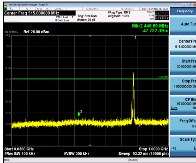
Band13-5MHz-QPSK-23230-1RB#0-Range1:30~1000MHz
